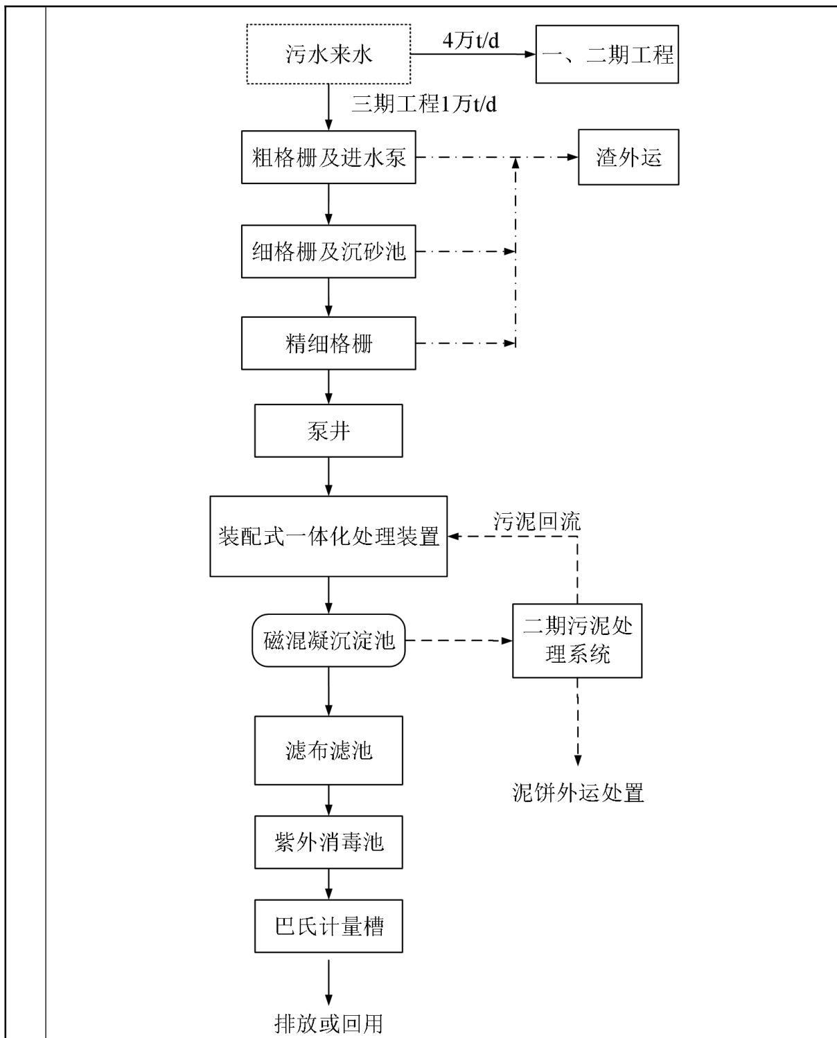
图 2-1 工艺流程图
