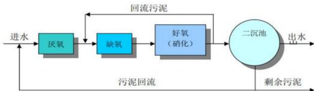
图 5.1-1 A 2 /O 工艺流程图
