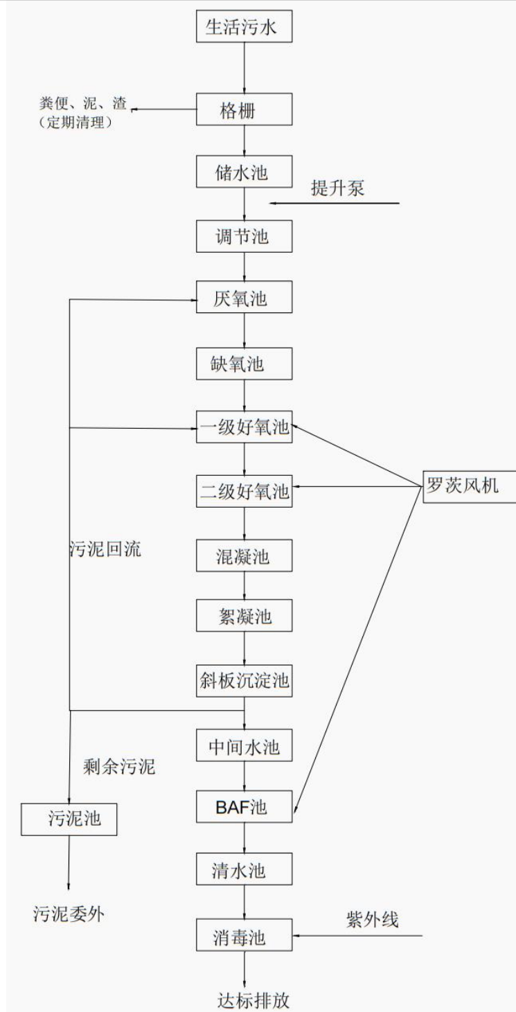
图 2-1 工艺流程框图
