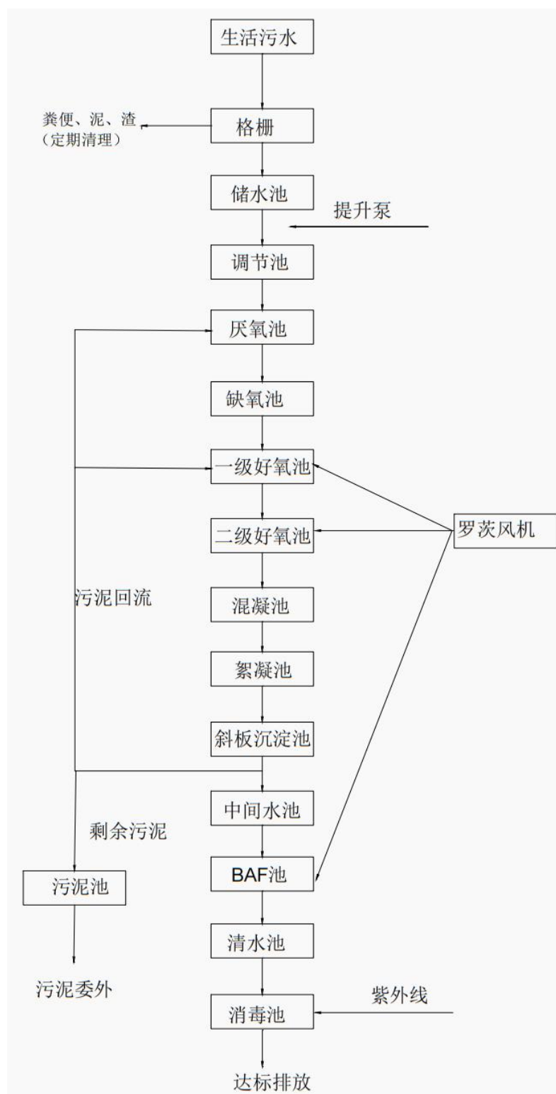
图 5.2-1 污水处理工艺流程图
