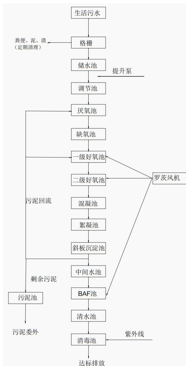
图 2-1 工艺流程框图
