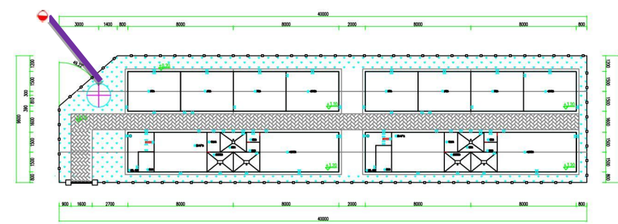
仙庵镇污水处理站(1) 平面布置图
