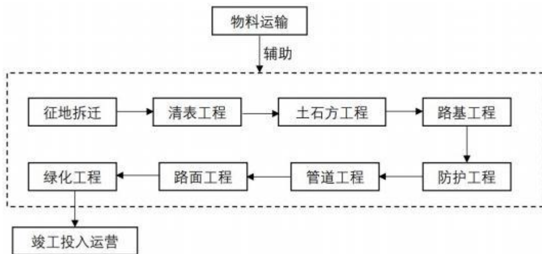
图2.4-1 施工工艺流程
