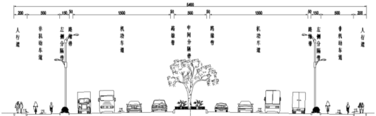
图2.2-1 路基标准横断面图
