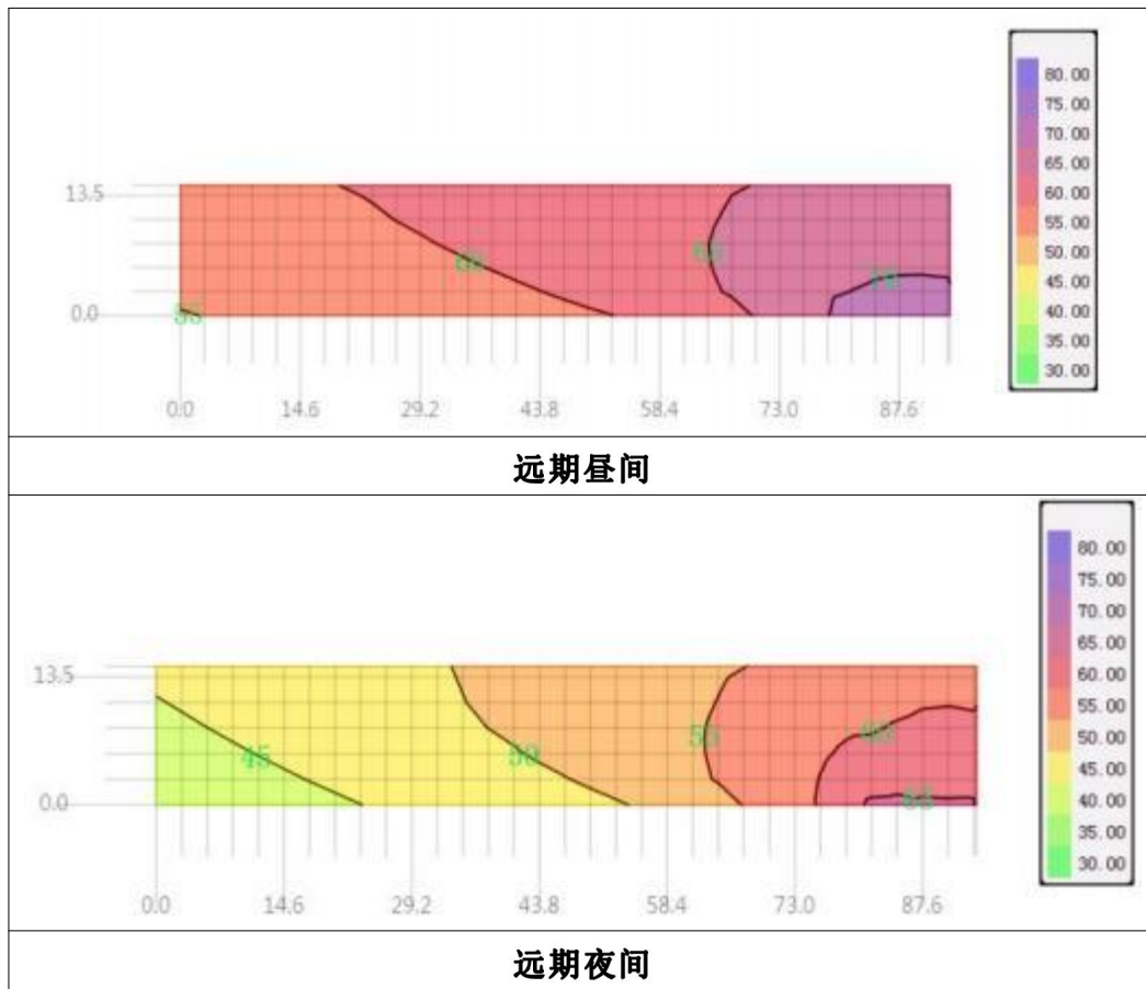
图5.2-2 沿线典型敏感点垂向网格等声级线图
