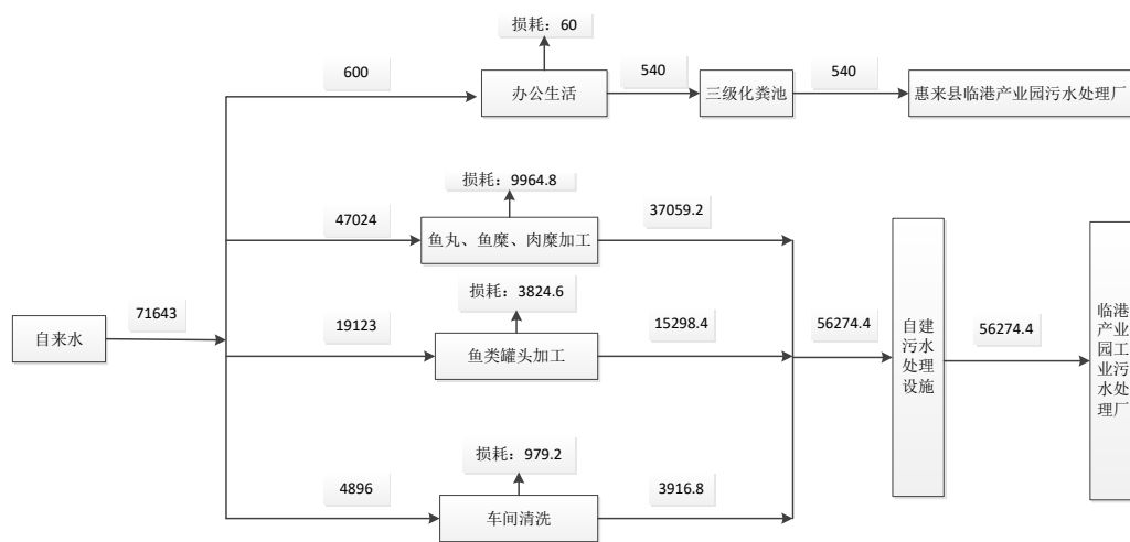
远期水平衡图
