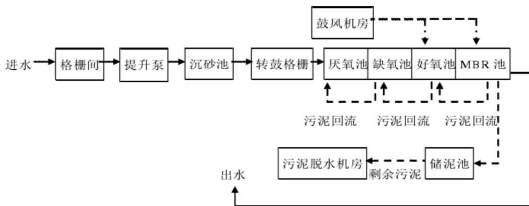
A/A/O 式 MBR 工艺流程图
