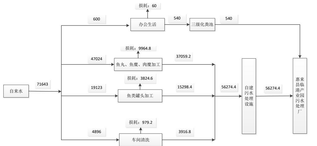
近期水平衡图
