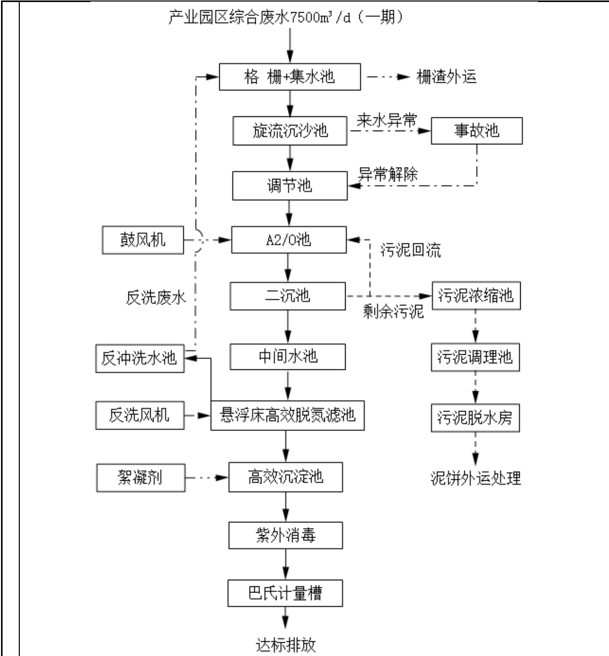
临港产业园污水处理厂工艺流程图
