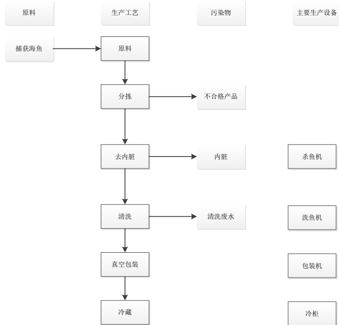
捕捞类冰鲜产品工艺流程
