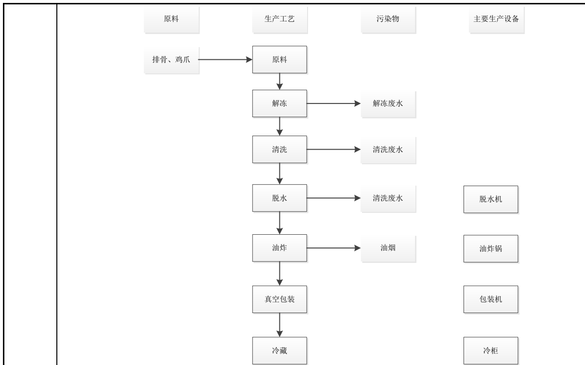
图 2-5 油炸食品生产工艺流程及产污节点图
