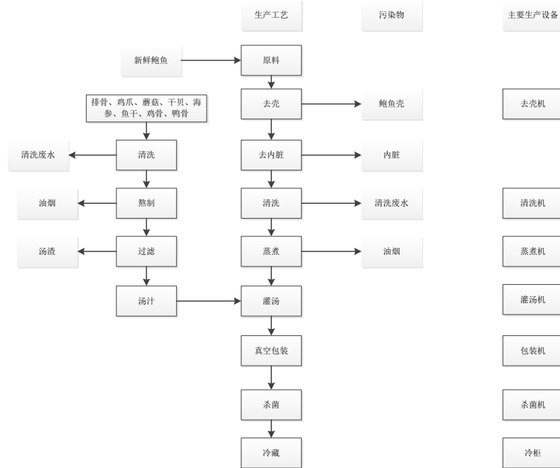
图 2-4 鲍鱼罐头生产工艺流程及产污节点图
