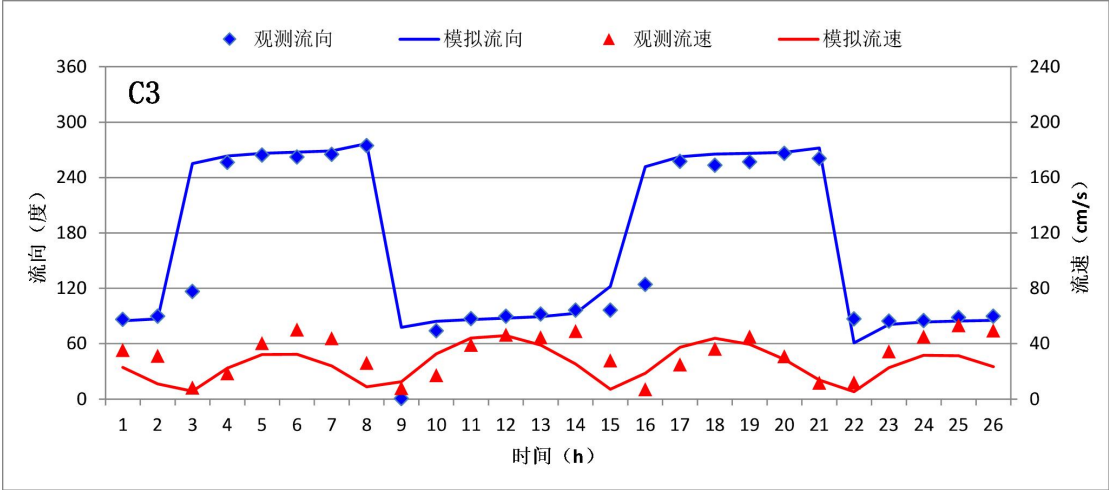
图 4.3.1-10 C3 站潮流验证曲线
