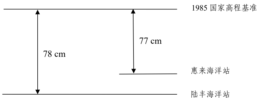
图 3.2.3-2 潮位站平均海面与 1985 国家高程基准面关系
