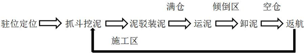
图2.3.1-2a 抓斗式挖泥工艺流程图
