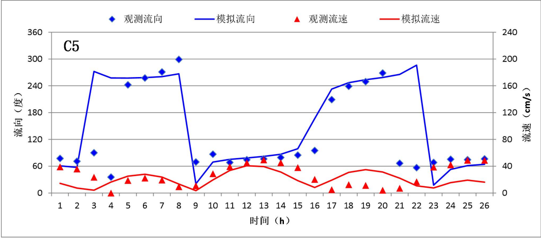
图 4.3.1-12 C5 站潮流验证曲线
