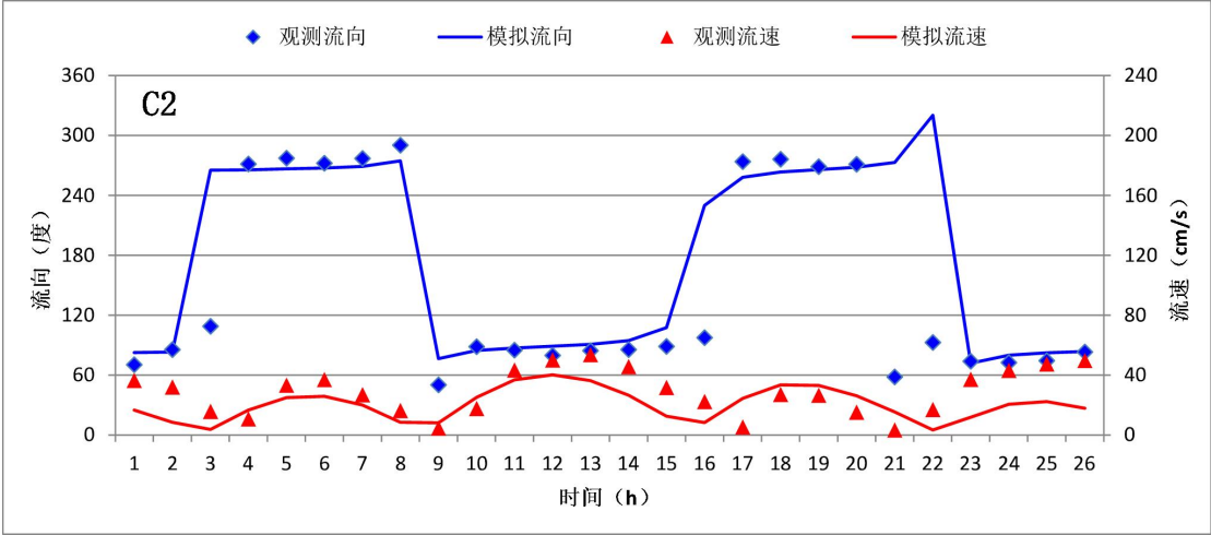
图 4.3.1-9 C2 站潮流验证曲线
