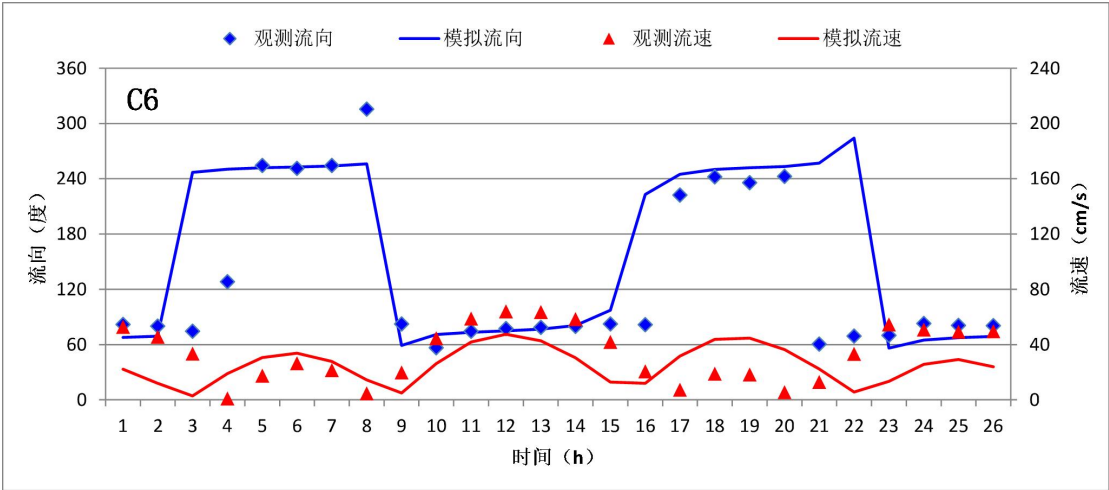
图 4.3.1-13 C6 站潮流验证曲线
