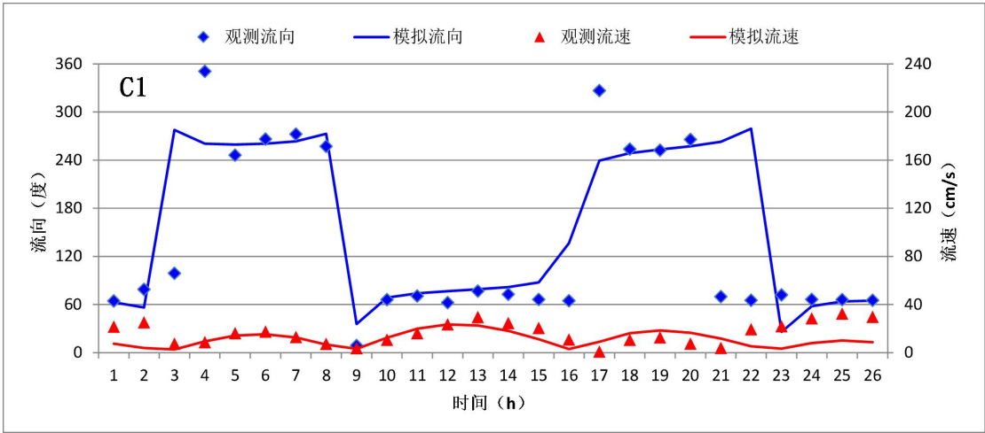
图 4.3.1-8 C1 站潮流验证曲线
