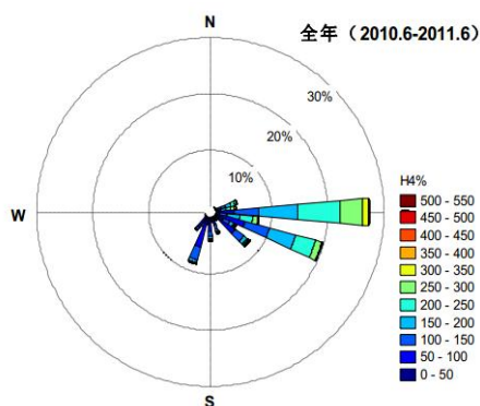
图 3.2.3-13 石碑山海域 2010 年 6 月~2011 年 6 月波浪玫瑰图
