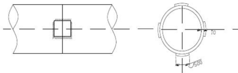
图 2.3.1-7 钢管桩接桩示意图
