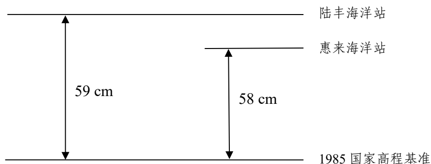
图 3.2.2-14 潮位站平均海面与 1985 国家高程基准面关系
