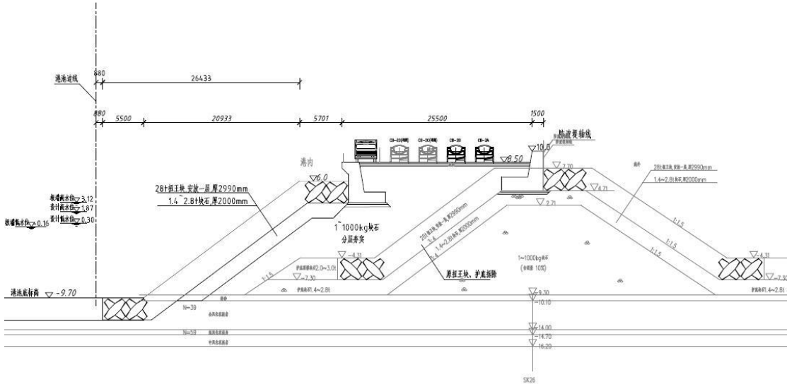
图 4.1.3-5 引桥根部斜坡堤加宽方案
