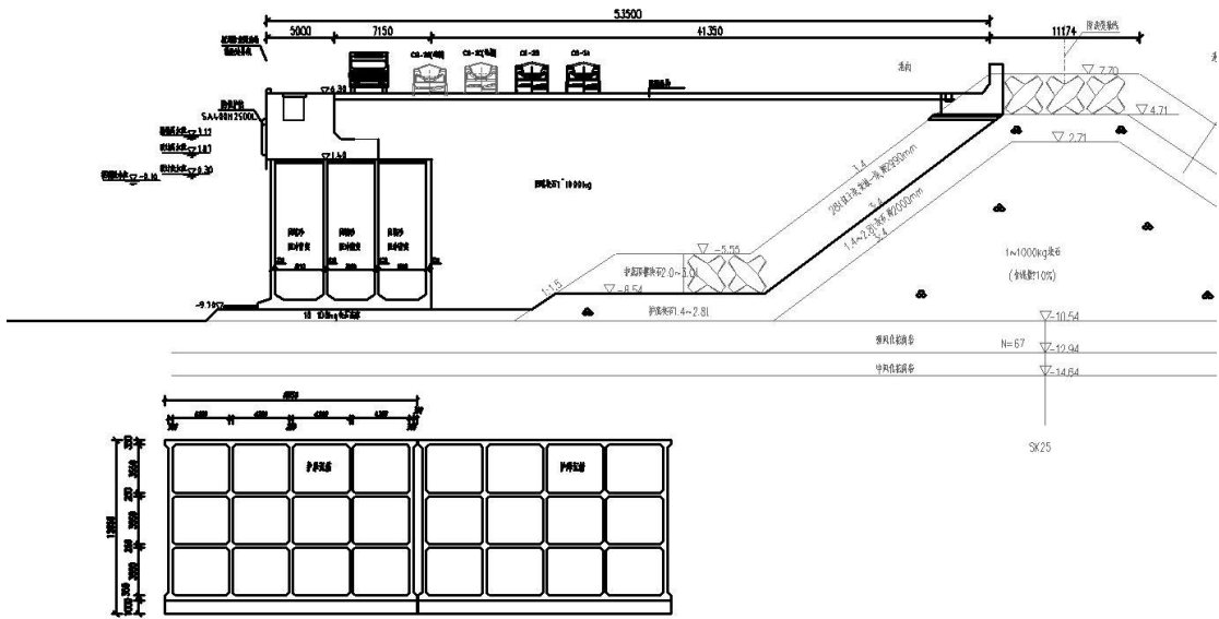
图 4.1.3-6 引桥根部沉箱加宽方案
