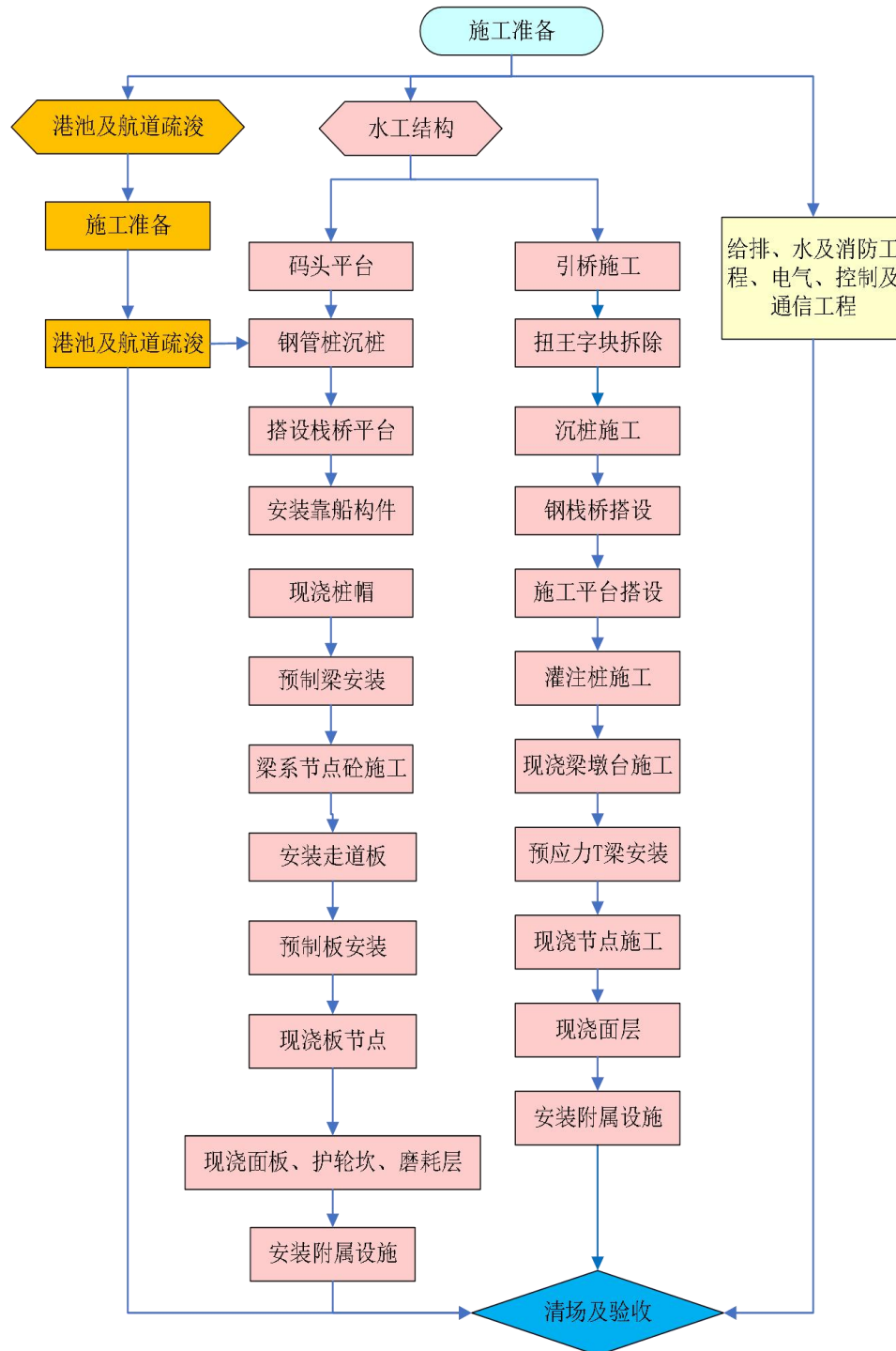
图 2.3-1 施工流程示意图
