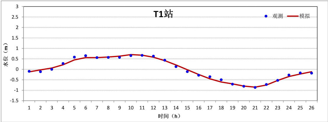
图 4.3.1-7 T1 站潮位验证曲线
