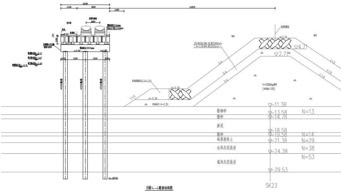
图 4.1.3-4 引桥结构断面图（方案二）
