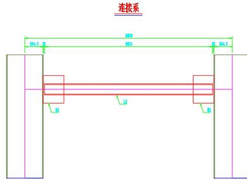
图 2.3.1-9 连接系安装示意图
