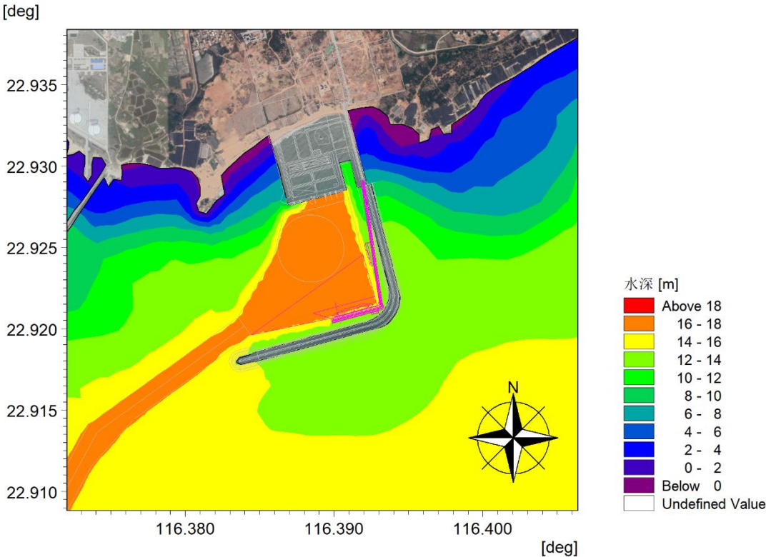
图 4.3.1-5 工程附近海域局部水深分布图（工程后）
