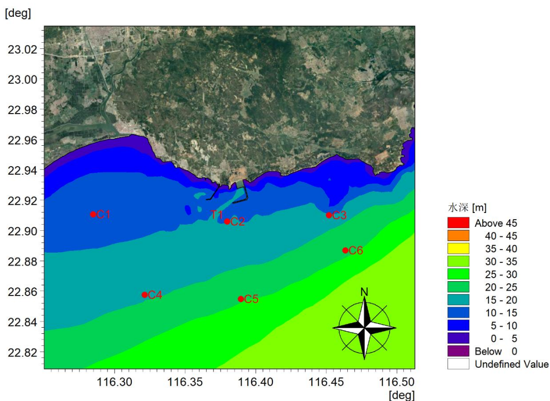
图 4.3.1-6 潮位(T1)、潮流(C1~C6)观测站位图
