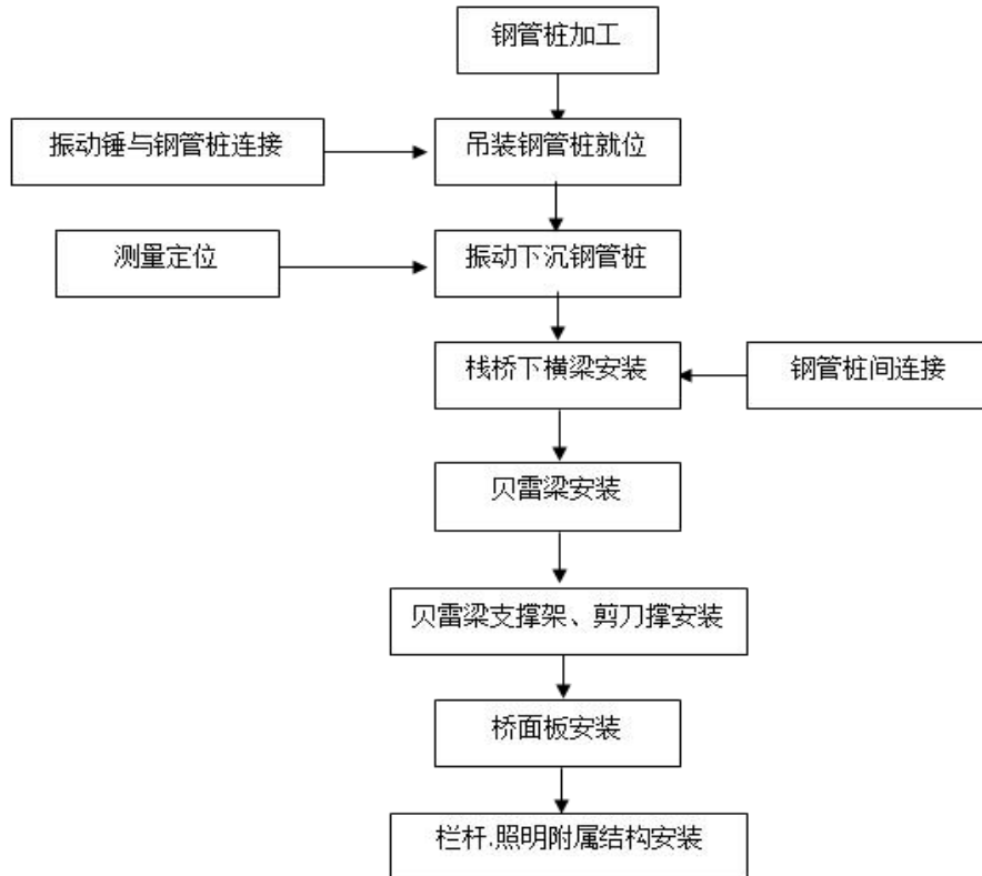
图 2.3.1-5 施工工艺流程图
