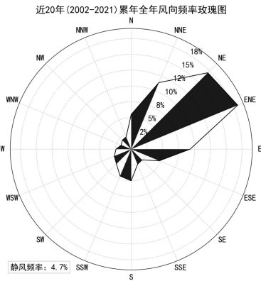
图 3.2.1-1 惠来气象站近 20 年（2002-2021）风向频率玫瑰图
