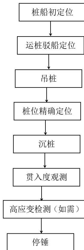
图 2.3.1-3 沉桩施工流程图
