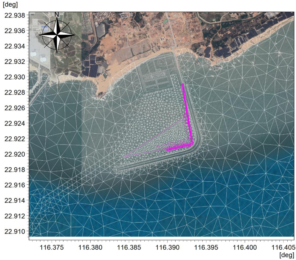
图 4.3.1-2 工程附近海域局部网格分布图
