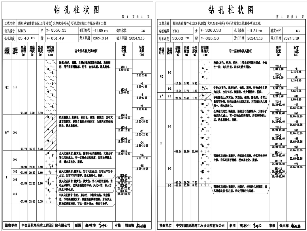
图 3.2.2-5 钻孔柱状图 2
