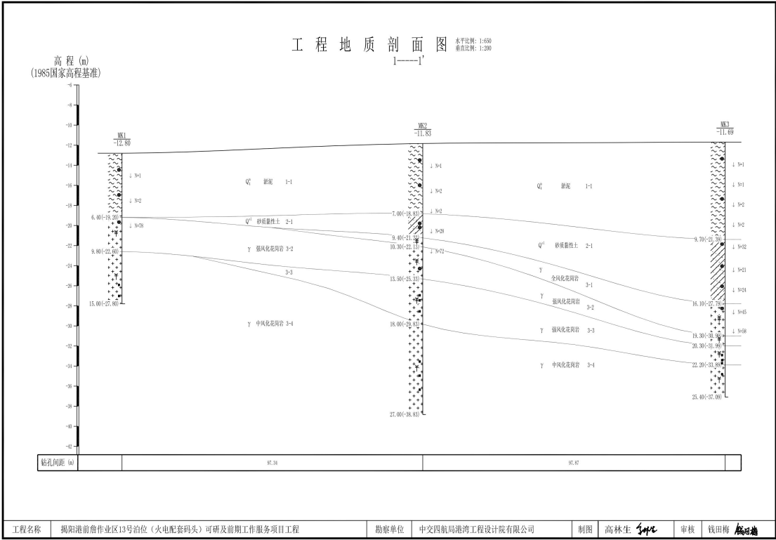
图 3.2.2-2 码头处地质剖面图
