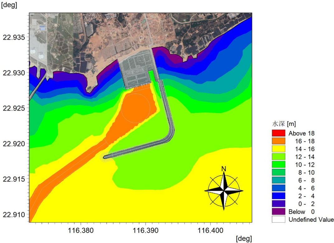
图 4.3.1-4 工程附近海域局部水深分布图（工程前）
