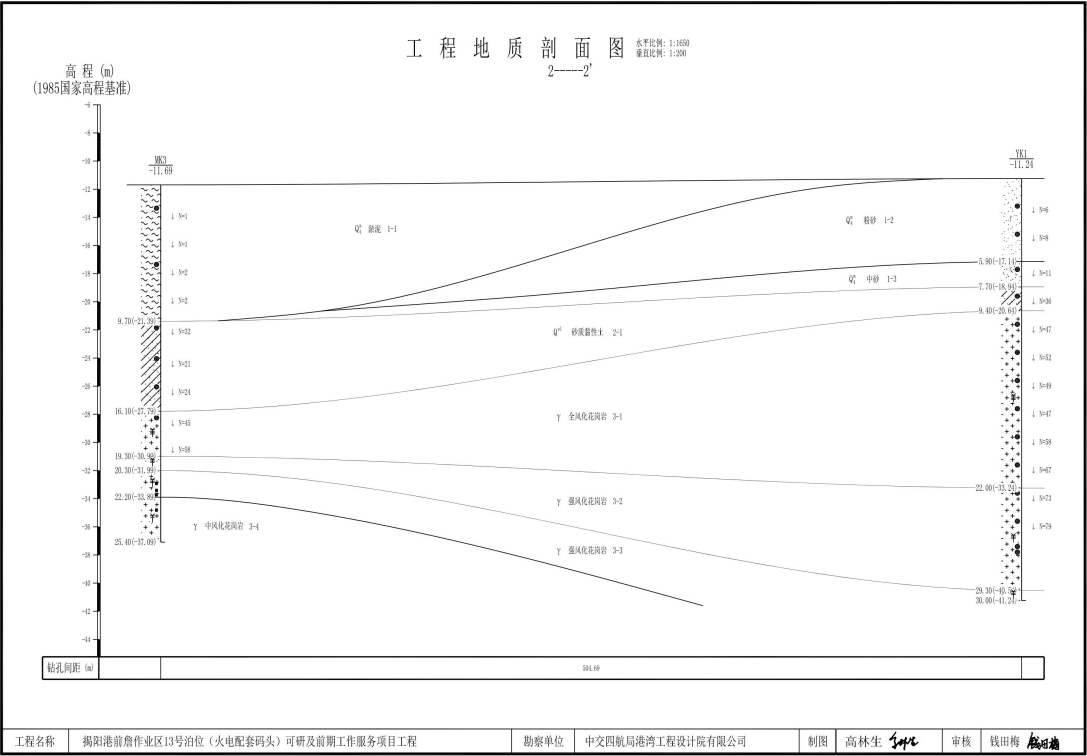
图 3.2.2-3 引桥处典型地质剖面图
