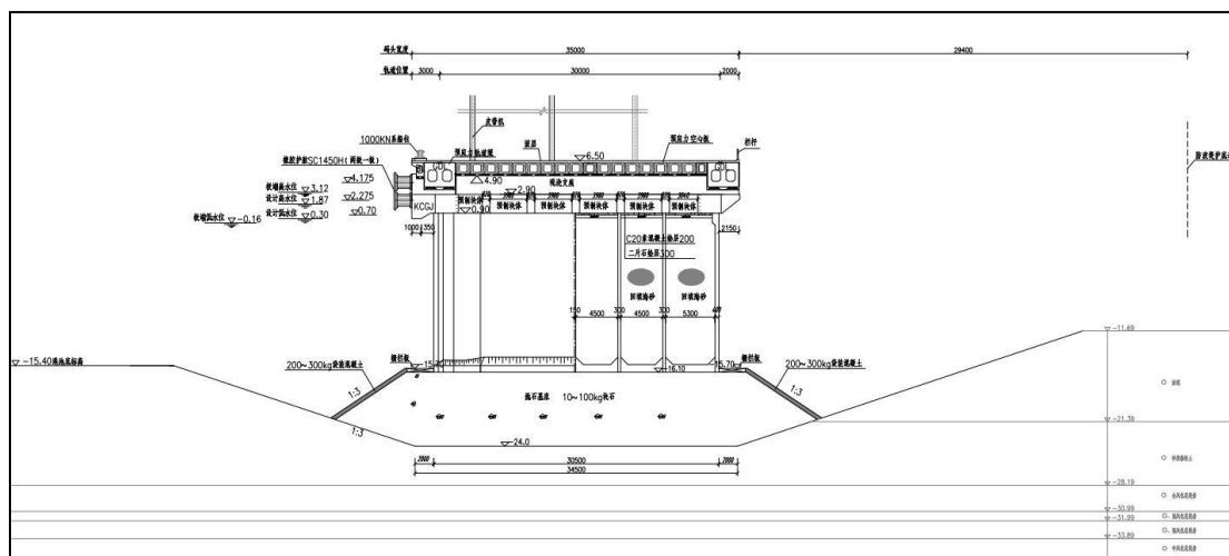
图 4.1.3-3 码头结构断面图 (方案二)
