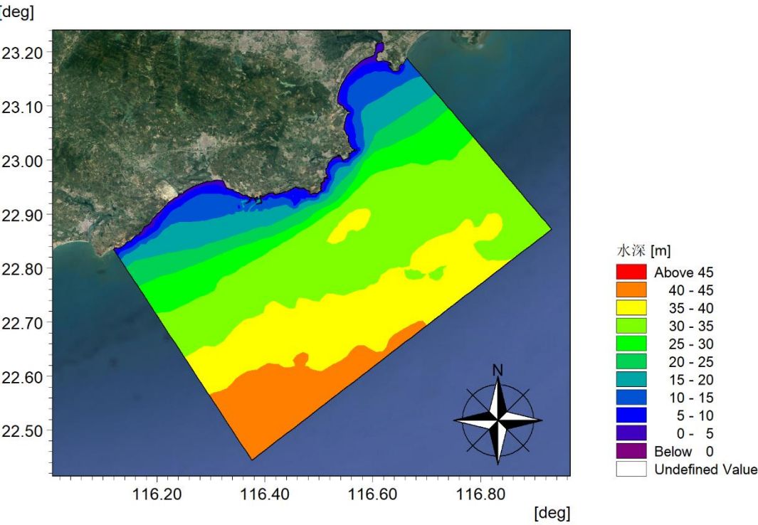
图 4.3.1-3 模型计算区域水深分布图
