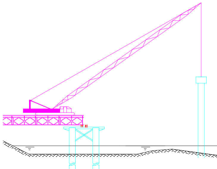
图 2.3.1-17 “钓鱼法”拔除钢管桩示意图
