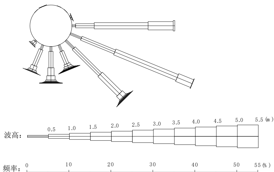
图 3.2.3-11 Hs 波浪玫瑰图 (2008 年 8 月~2009 年 7 月)
