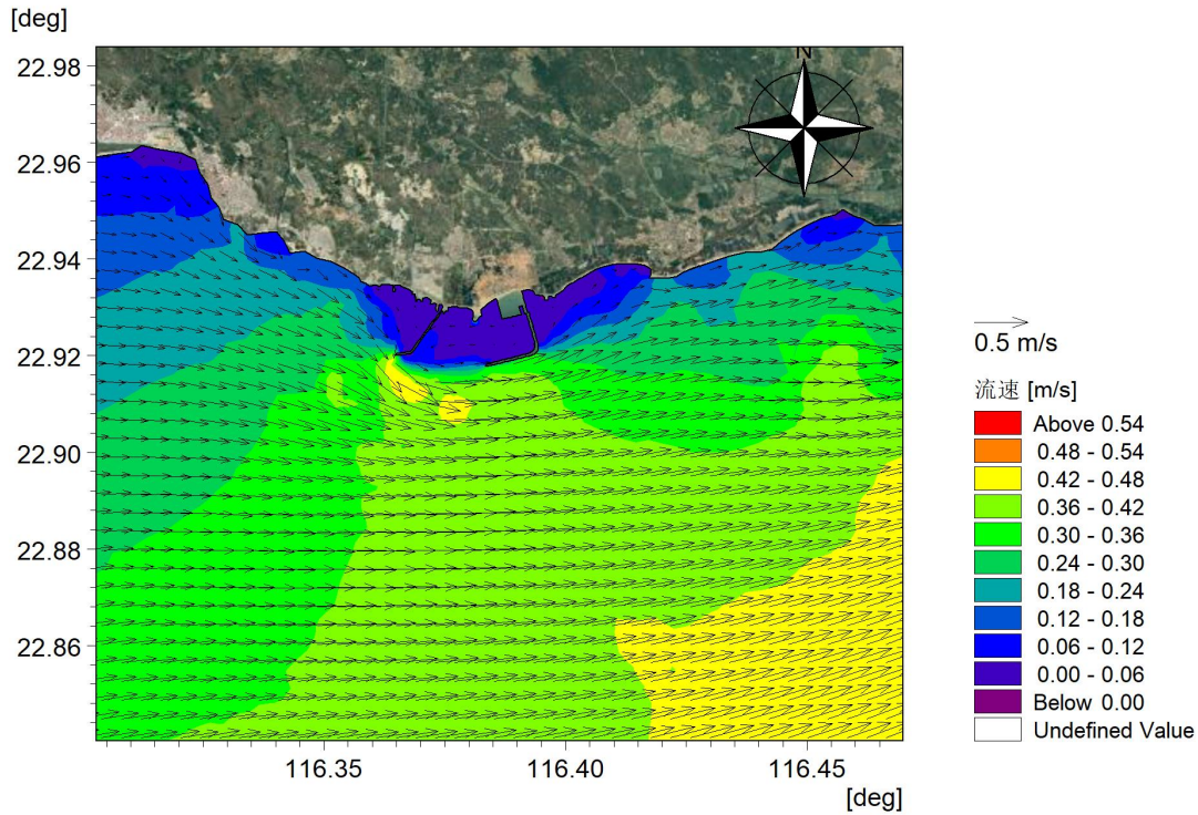
图 4.3.1-14 模拟的大区域潮流场分布（涨急时，大潮期）
