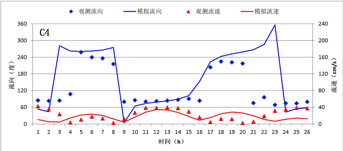
图 4.3.1-11 C4 站潮流验证曲线
