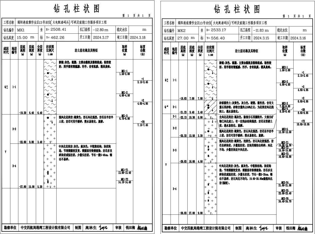
图 3.2.2-4 钻孔柱状图 1
