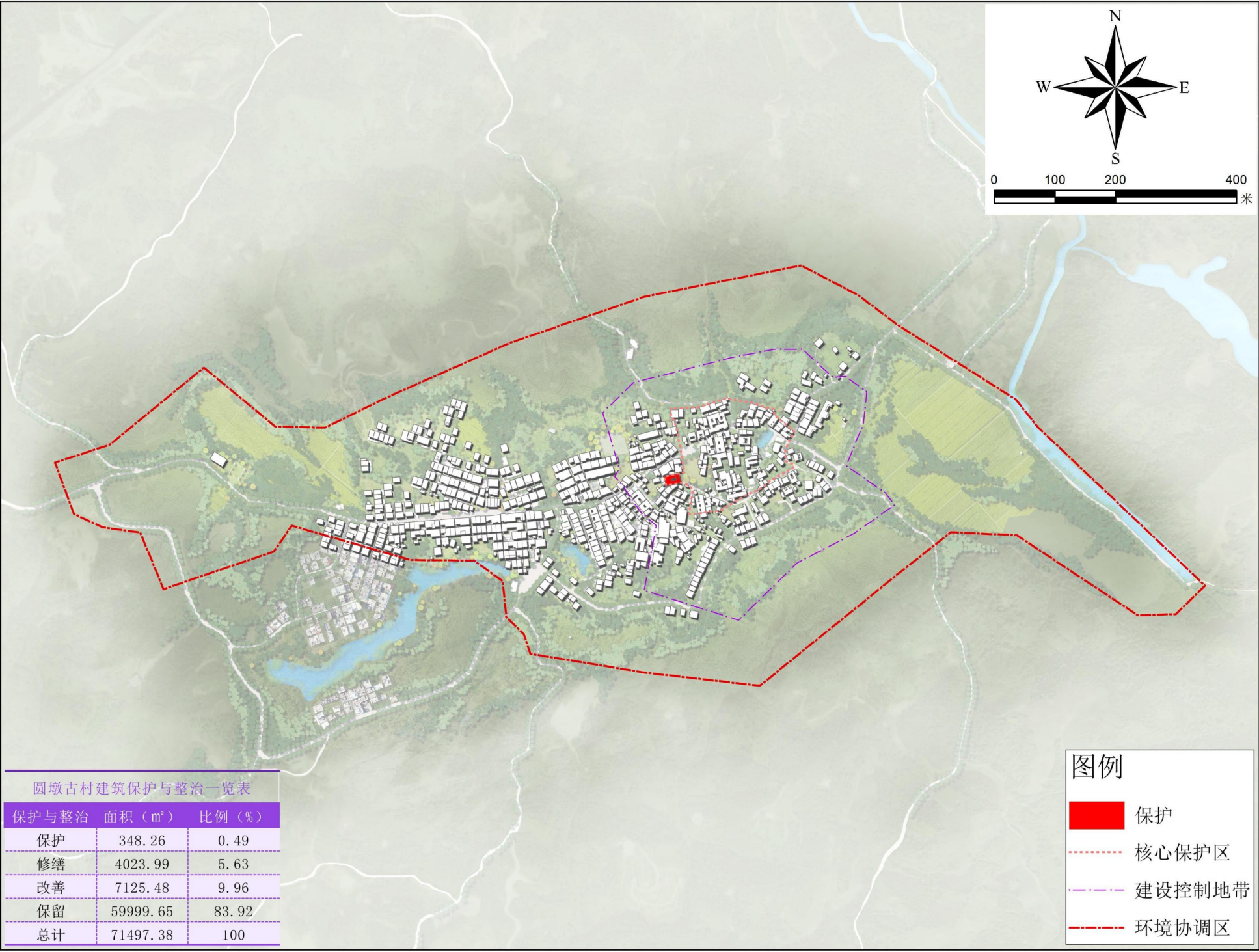
图3-7 保护建筑分布图
