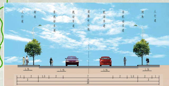
主要道路横断面
