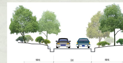
次要道路横断面
