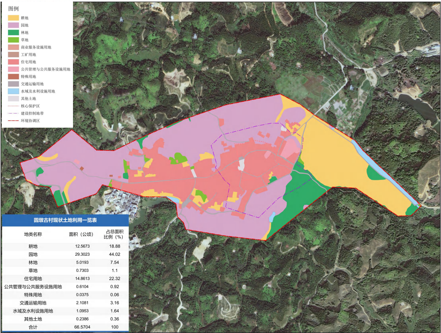
图2-11 土地利用现状图
