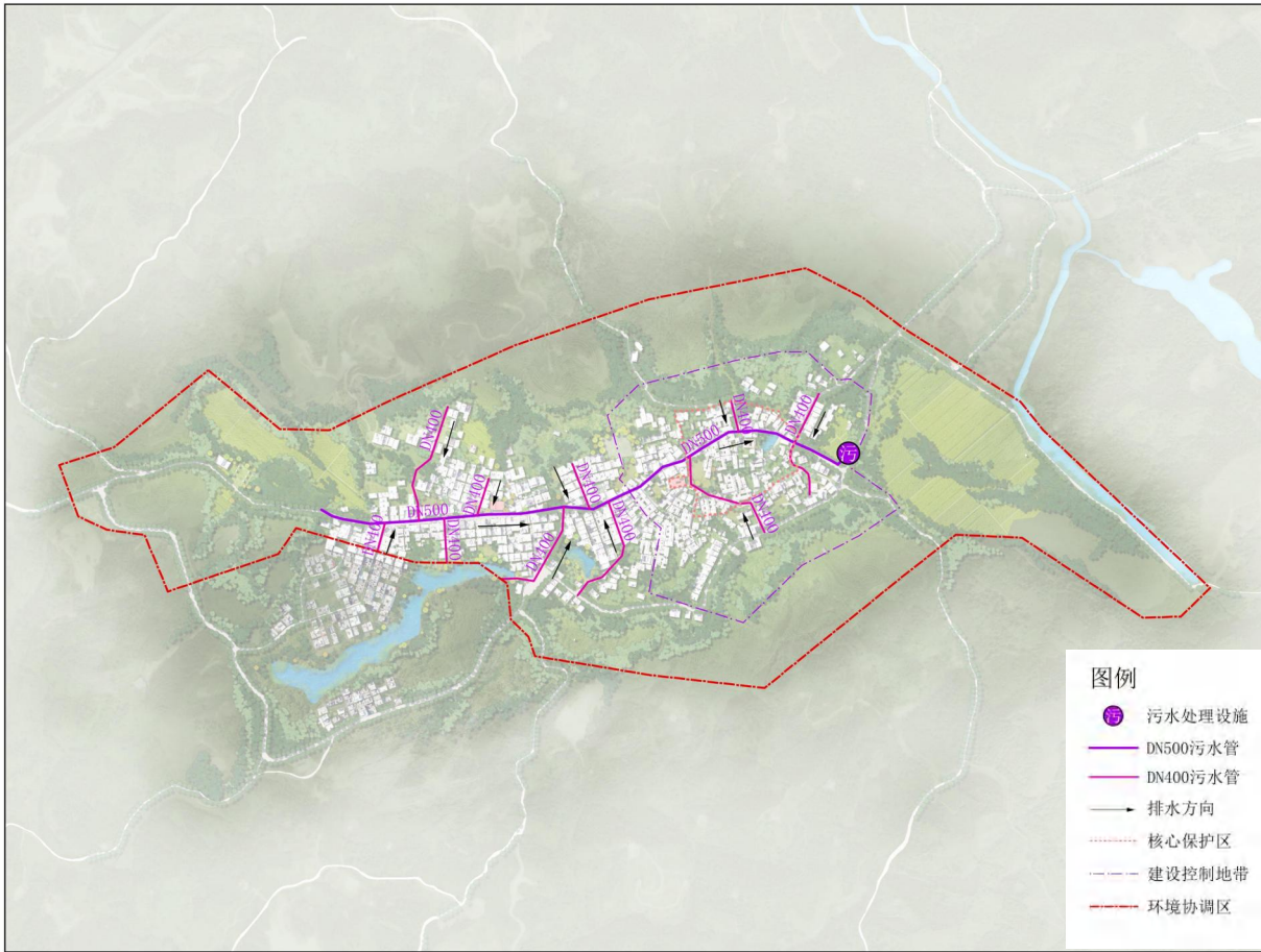
图4-14 污水工程规划图
