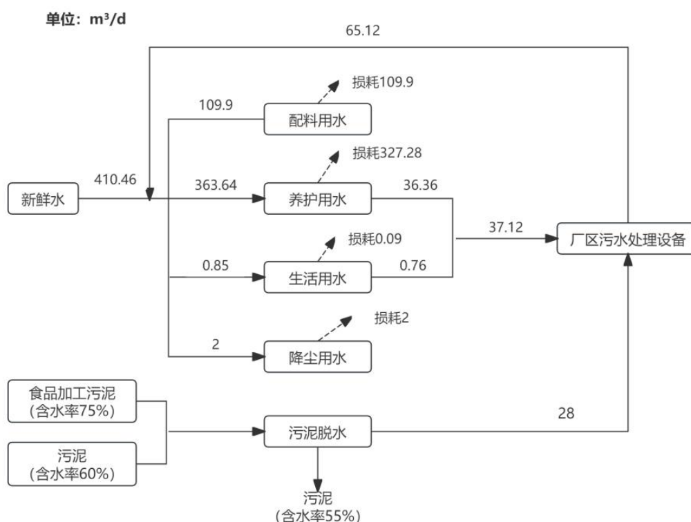
图 4-1 水平衡图
