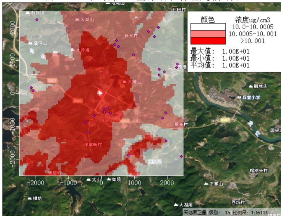
图 5.2-26 正常工况下 HCl 叠加后日平均质量浓度分布图
