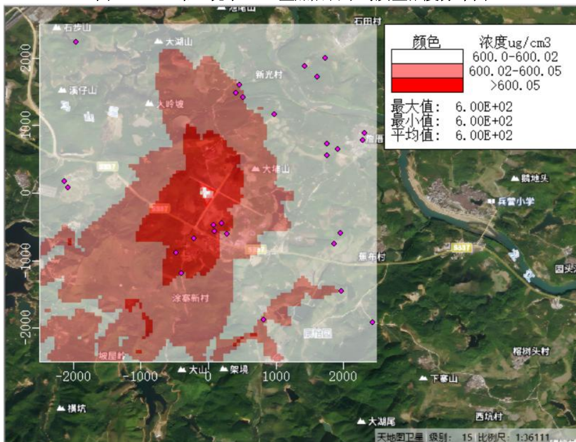
图 5.2-28 正常工况下 CO 叠加后日平均质量浓度分布图
