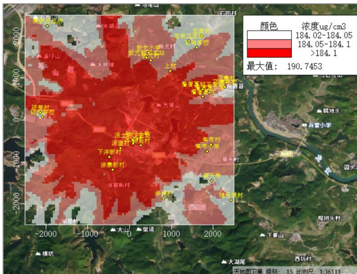
图 5.2-27 正常工况下 TSP 叠加后日平均质量浓度分布图
