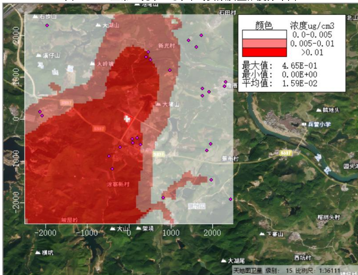
图5.2-20 正常工况下NO x 年平均贡献质量浓度分布图
