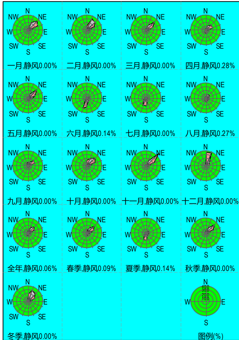
图 5.2-6 风频玫瑰图
