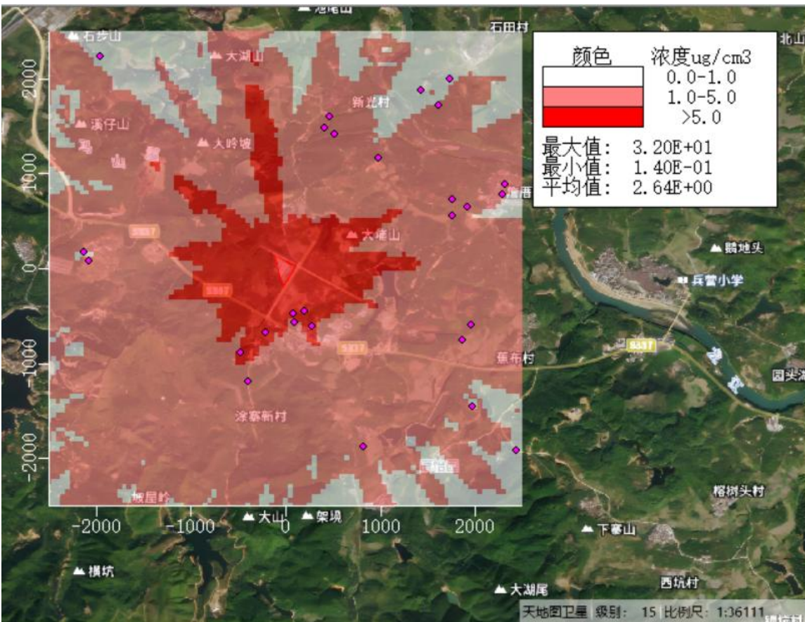
图5.2-34 非正常工况下TSP 1小时平均贡献质量浓度分布图
