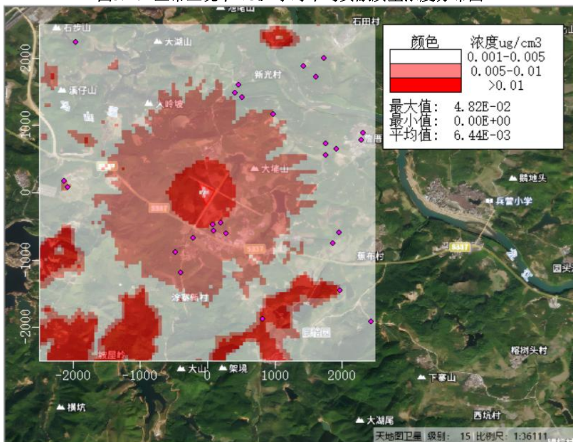
图5.2-10 正常工况下HCl 1小时平均贡献质量浓度分布图
