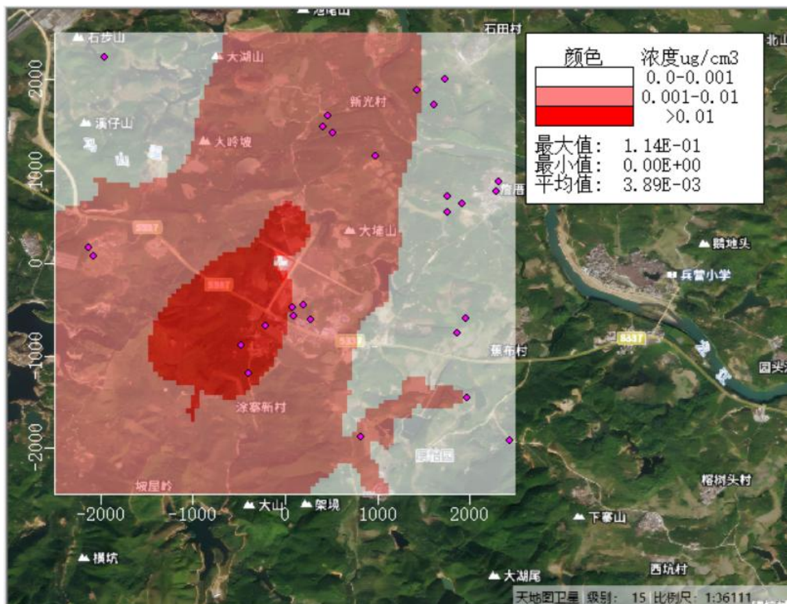
图5.2-19 正常工况下SO 2 年平均贡献质量浓度分布图
