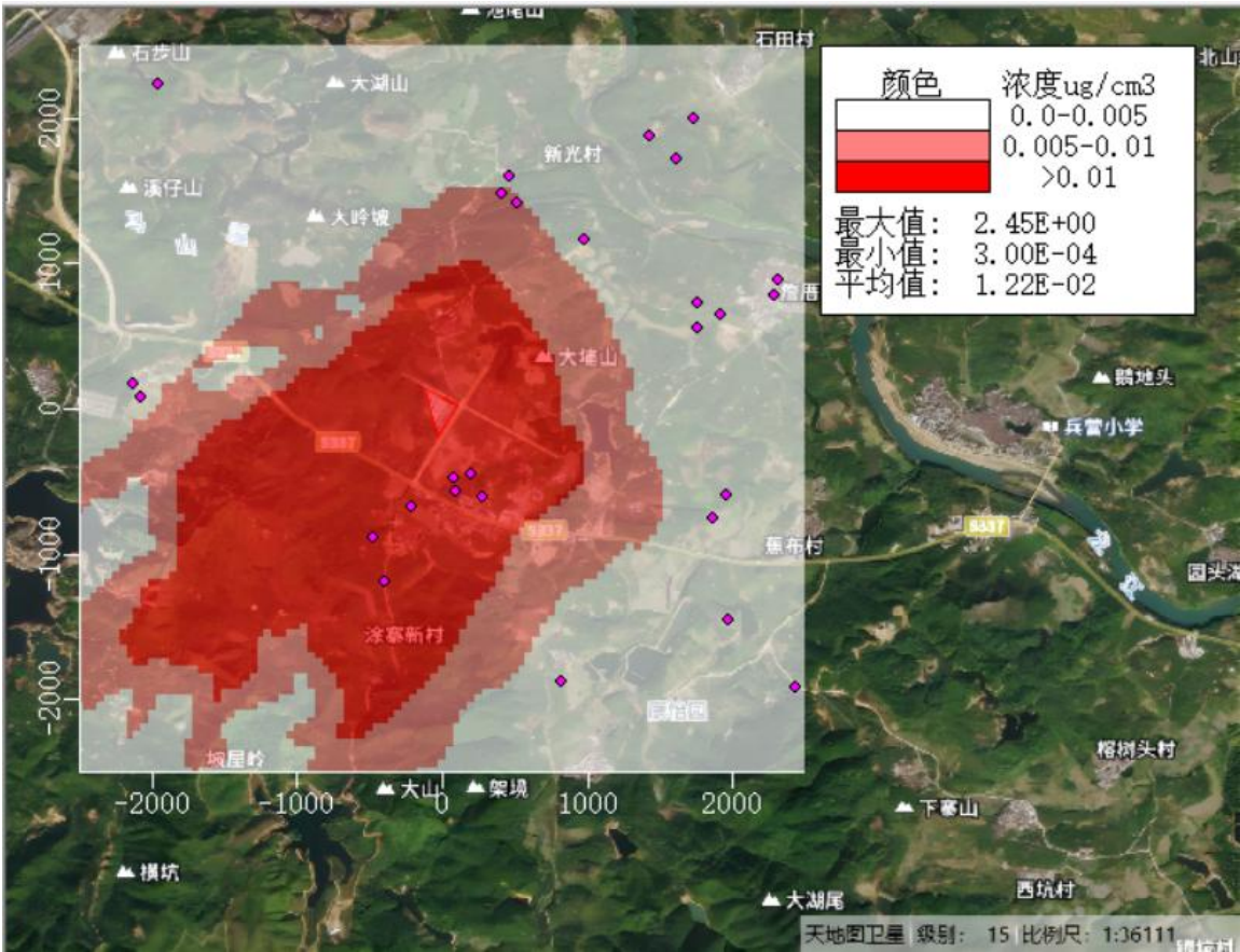
图5.2-21 正常工况下TSP年平均贡献质量浓度分布图
