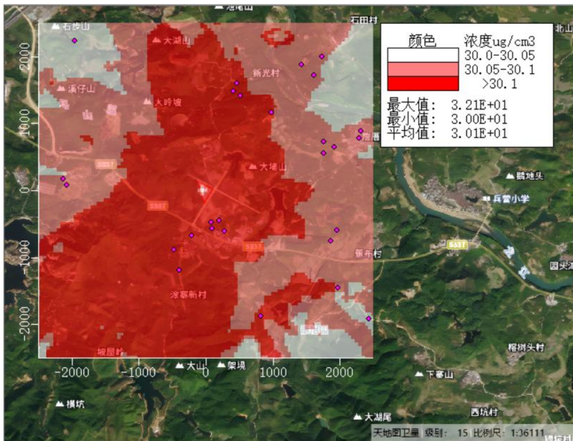
图 5.2-25 正常工况下 NO x 叠加后日平均质量浓度分布图
