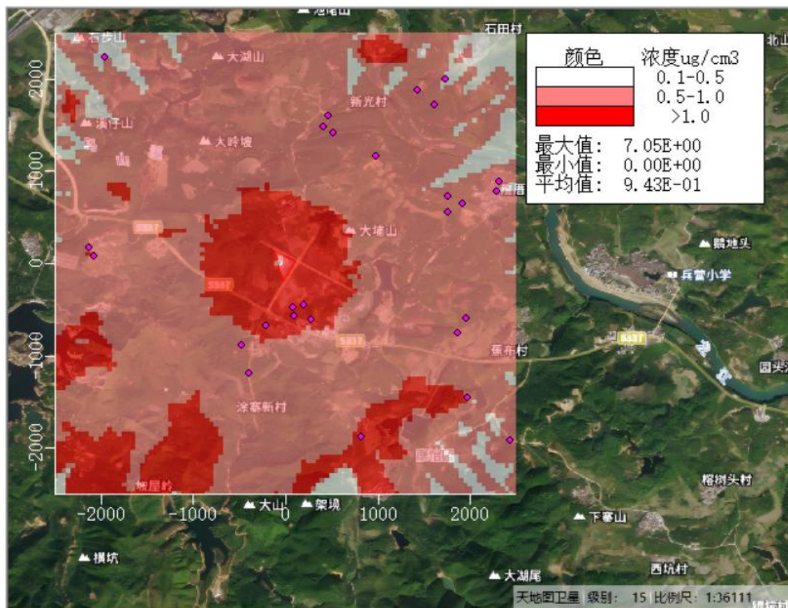
图5.2-9 正常工况下NO x 1小时平均贡献质量浓度分布图
