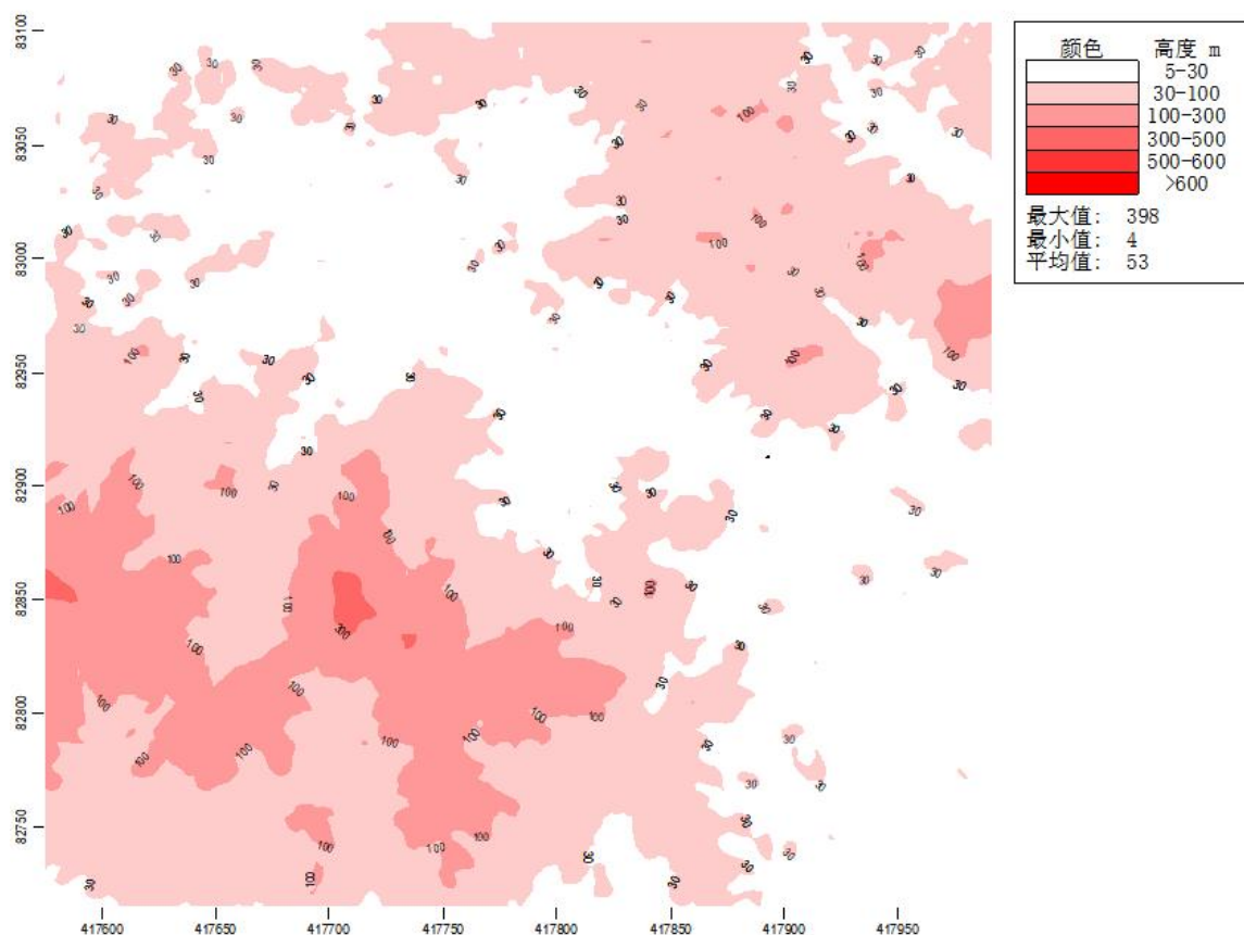
图5.2-7 预测区域地形特征图
