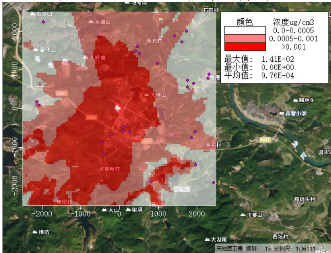
图5.2-16 正常工况下HCl日平均贡献质量浓度分布图
