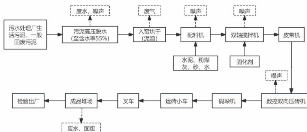
图 3.2-1 轨道窑生产线工艺流程图
