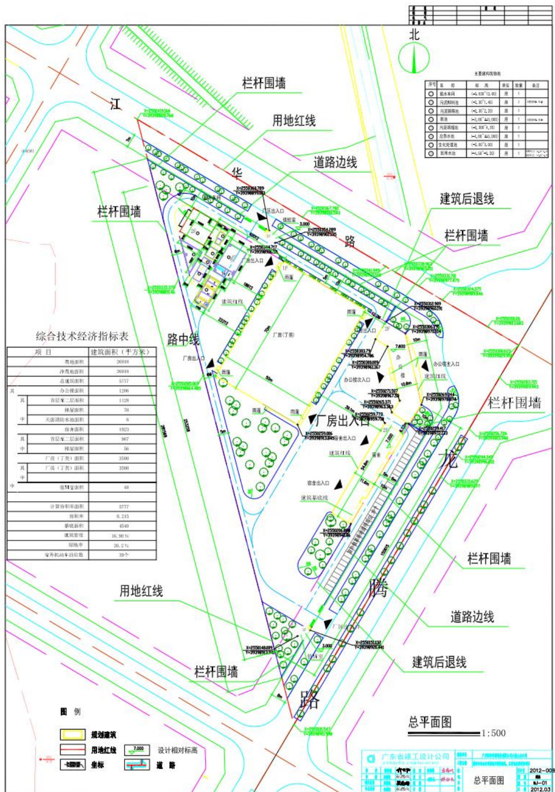
附图六 本扩建项目平面布置图
