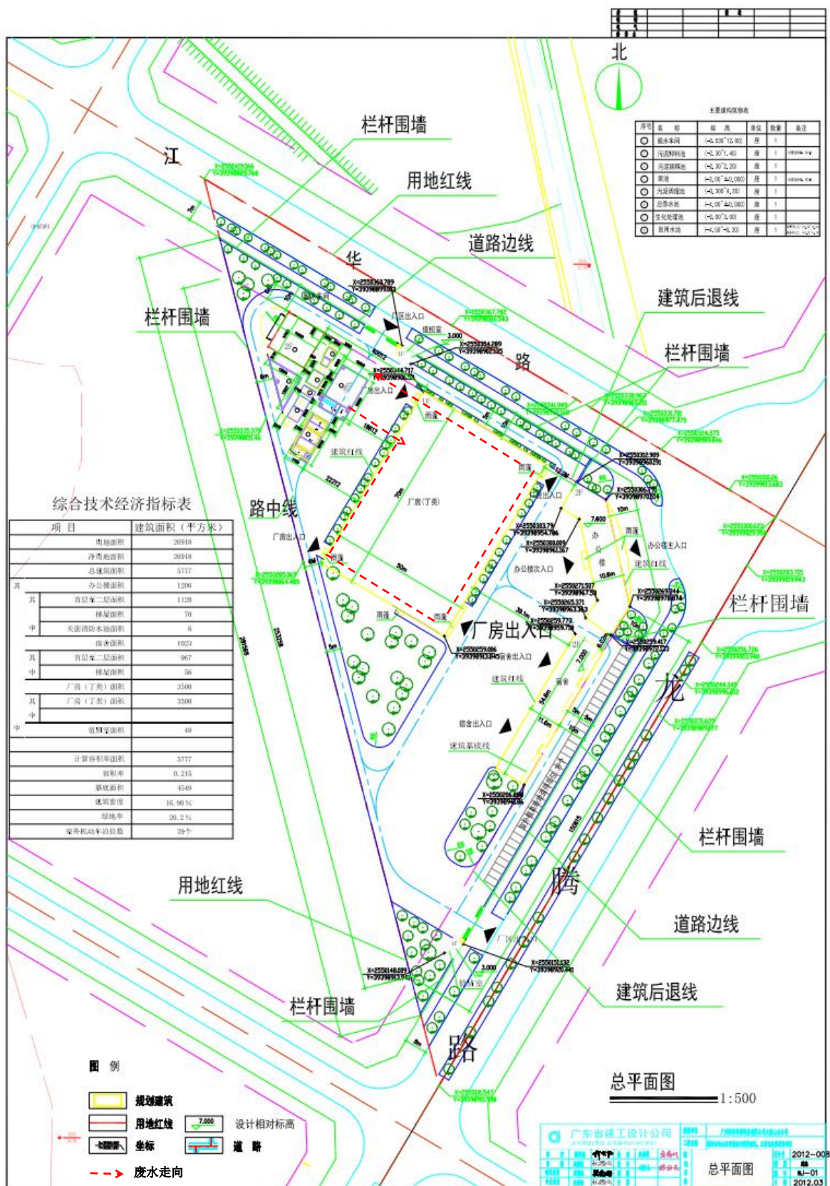
附图十一 本扩建项目废水走向图
