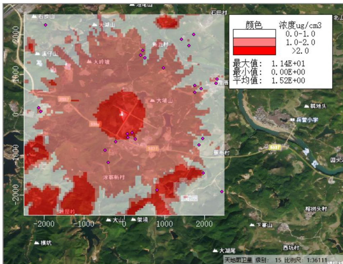
图5.2-32 非正常工况下SO 2 1小时平均贡献质量浓度分布图
