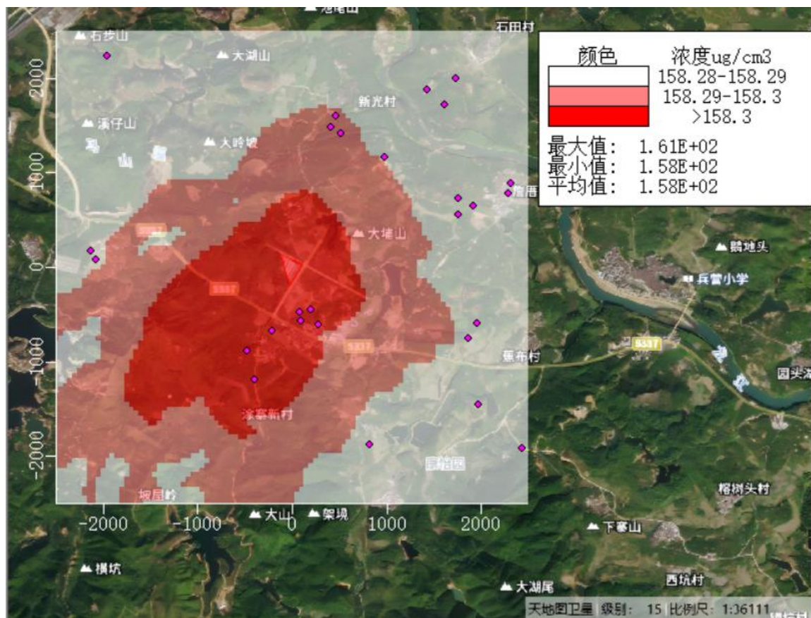
图 5.2-31 正常工况下 TSP 叠加后年平均质量浓度分布图
