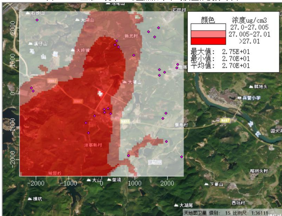
图 5.2-30 正常工况下 NO x 叠加后年平均质量浓度分布图
