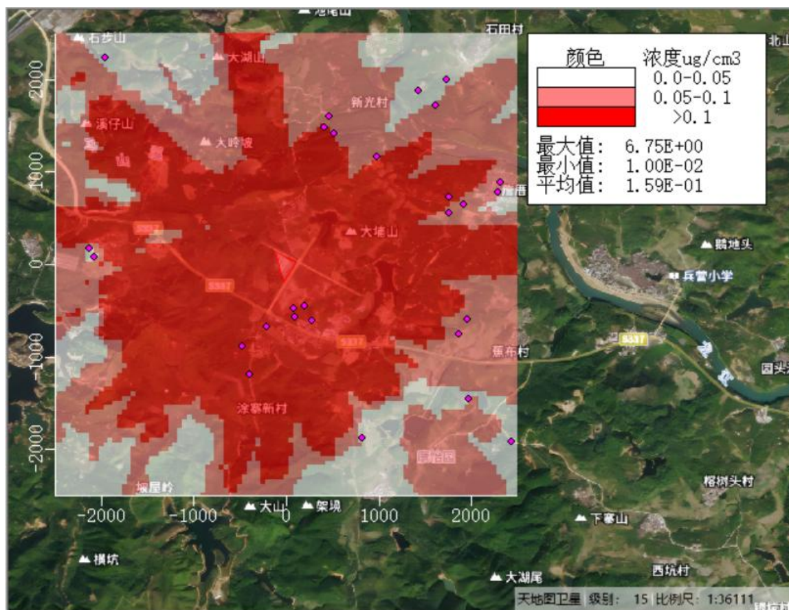
图5.2-17 正常工况下TSP日平均贡献质量浓度分布图
