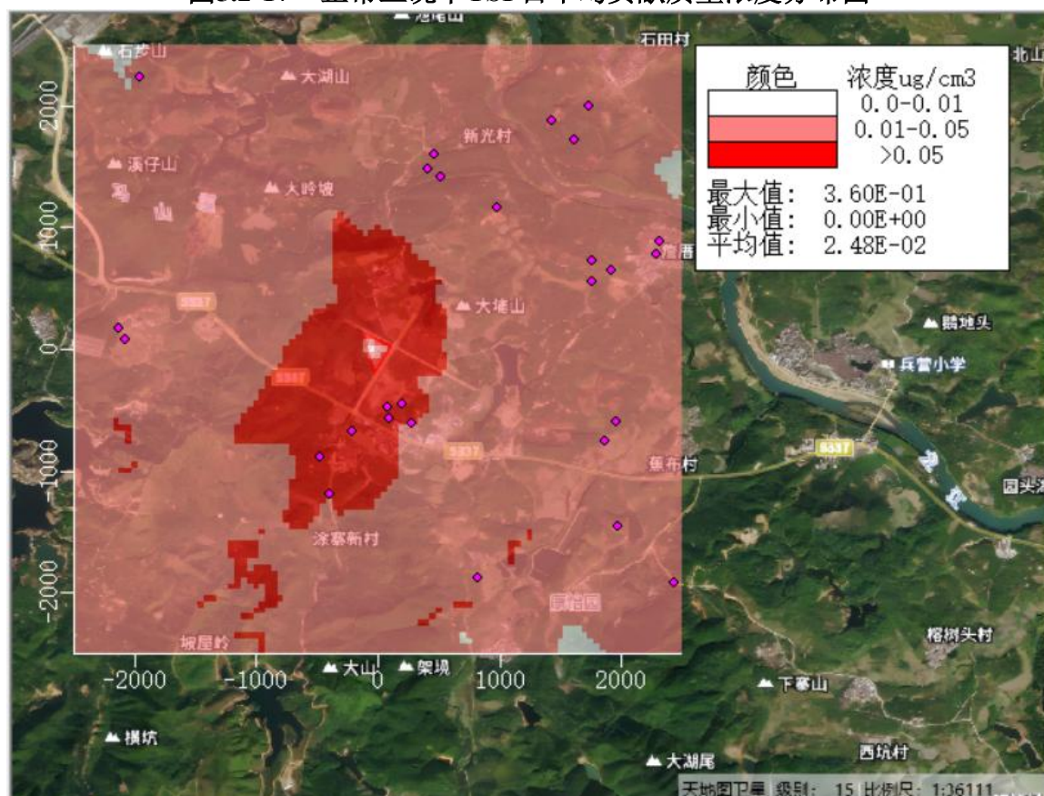
图5.2-18 正常工况下CO日平均贡献质量浓度分布图
