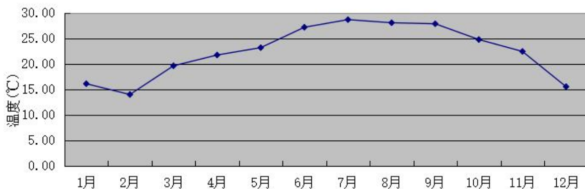
图 5.2-2 年平均温度的月变化图
