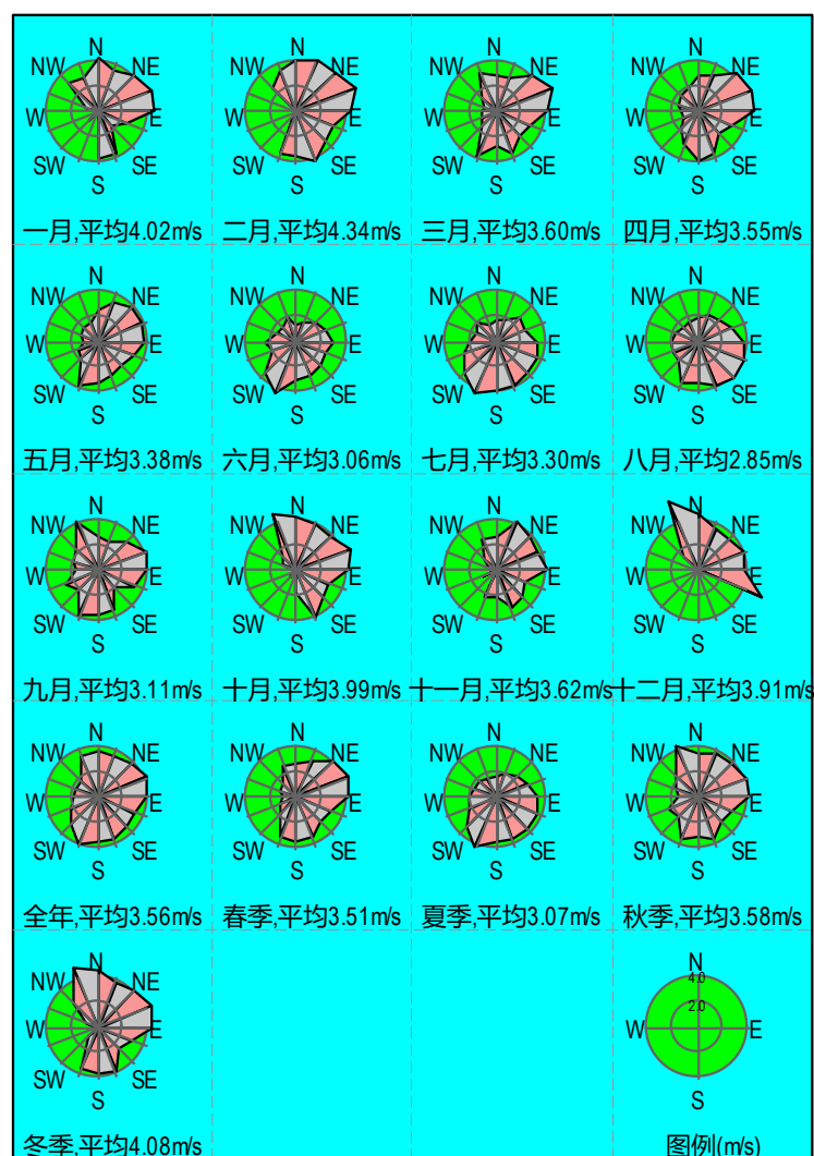
图 5.2-5 风速玫瑰图
