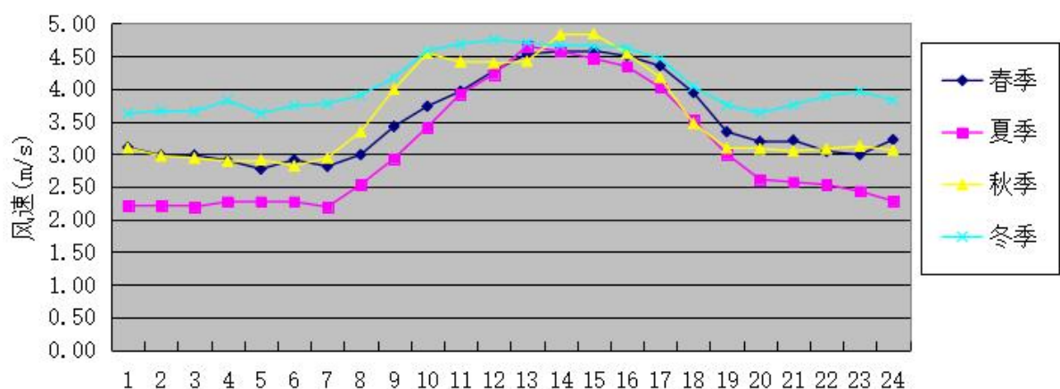
图 5.2-4 季小时平均风速的日变化图
