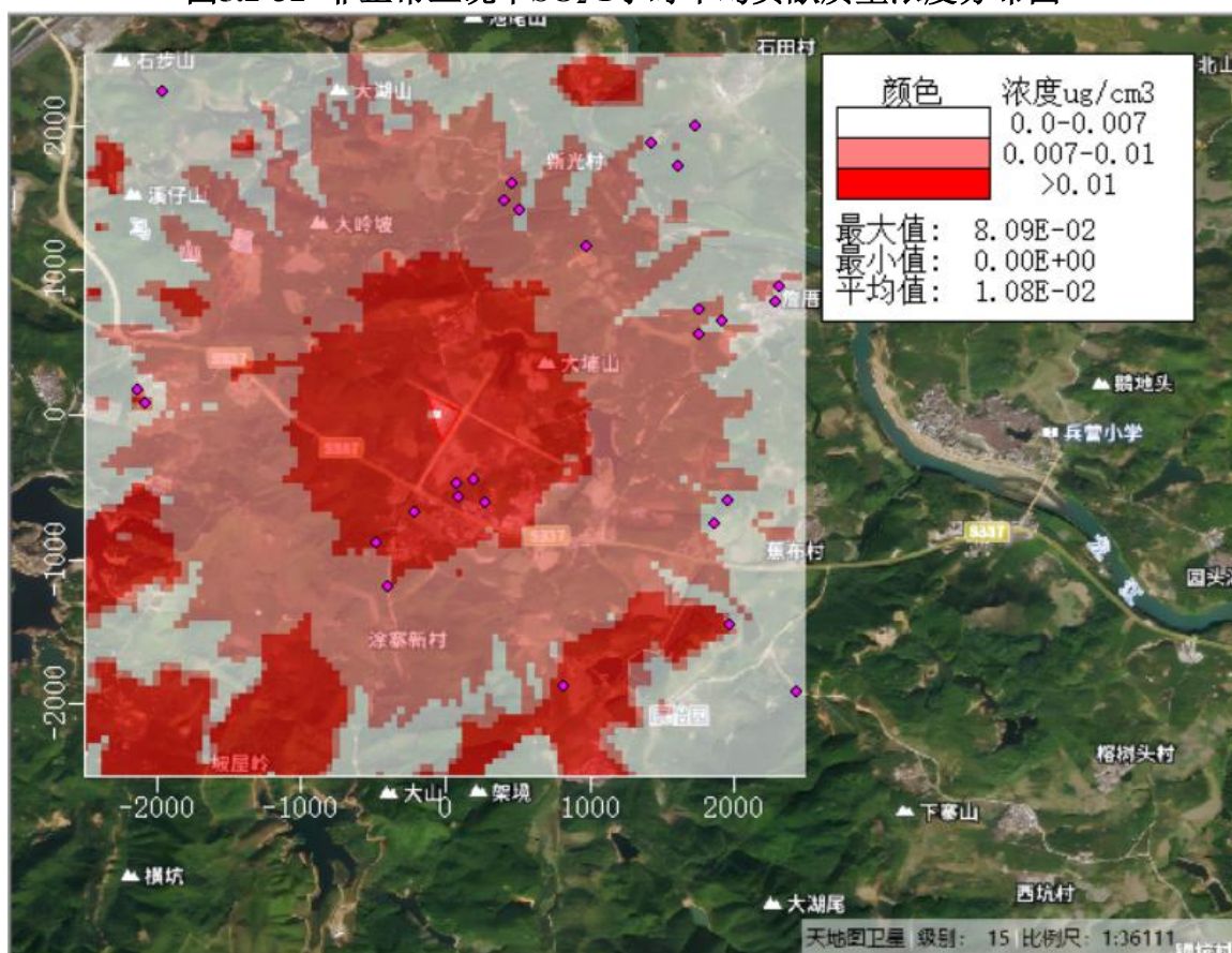
图5.2-33 非正常工况下HCl 1小时平均贡献质量浓度分布图
