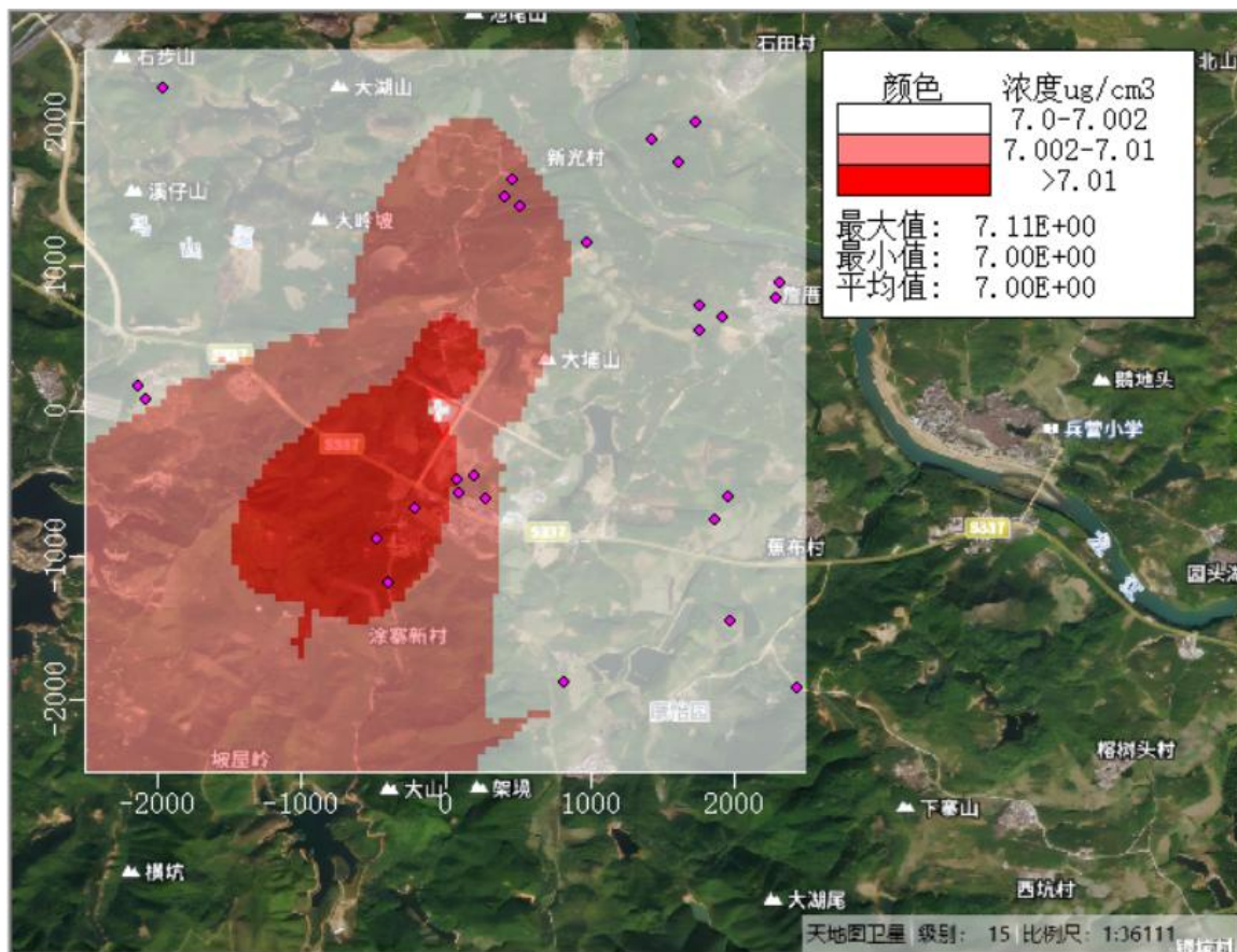
图 5.2-29 正常工况下 SO 2 叠加后年平均质量浓度分布图
