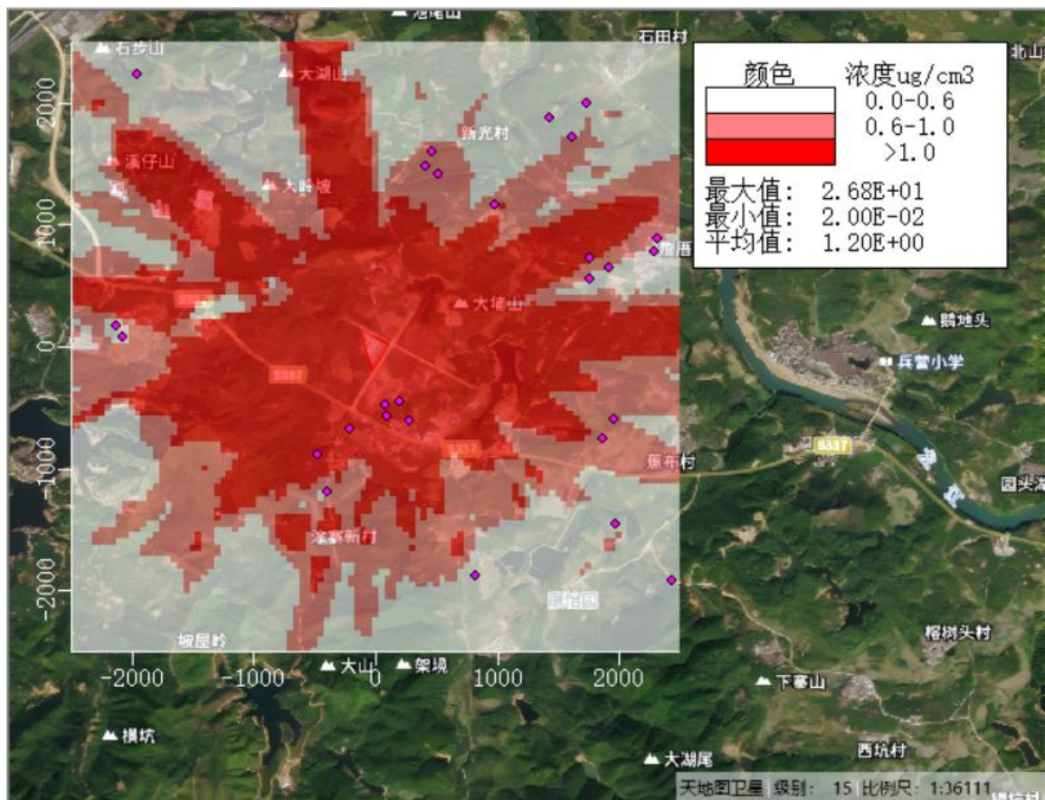
图5.2-13 正常工况下NH 3 1小时平均贡献质量浓度分布图
