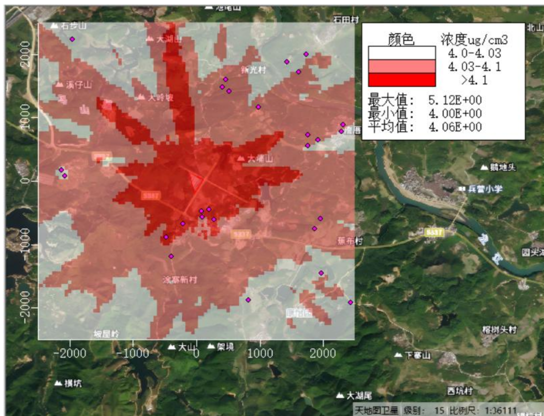
图 5.2-22 正常工况下 H 2 S 叠加后 1 小时平均质量浓度分布图
