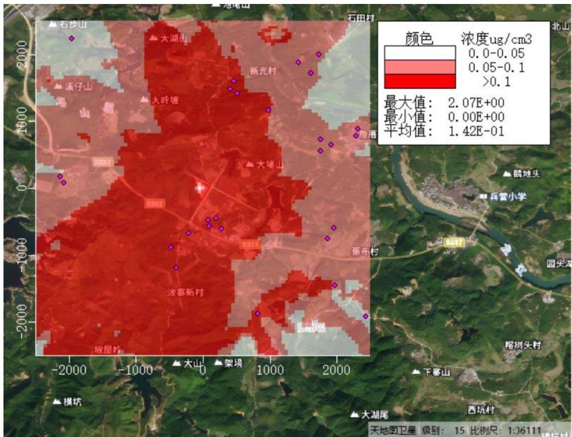
图5.2-15 正常工况下NO x 日平均贡献质量浓度分布图
