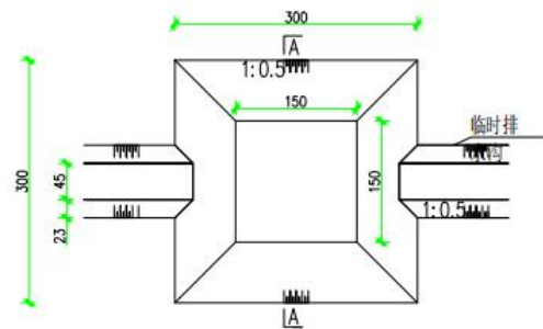
沉沙池平面布置图 1:50
