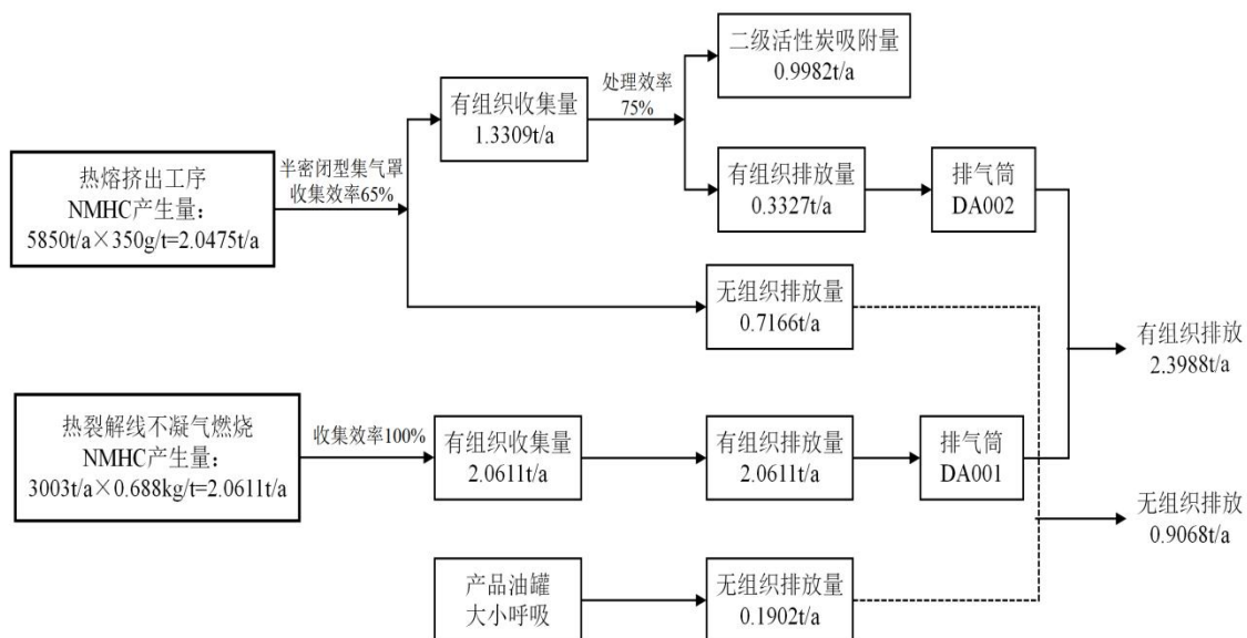
图2-1 VOCs物料平衡图
