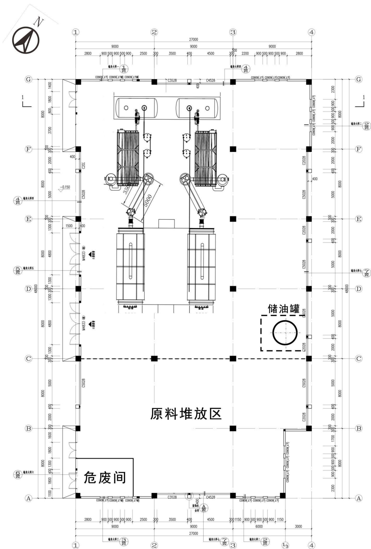
附图 2-3 项目厂房 C 平面布置图
