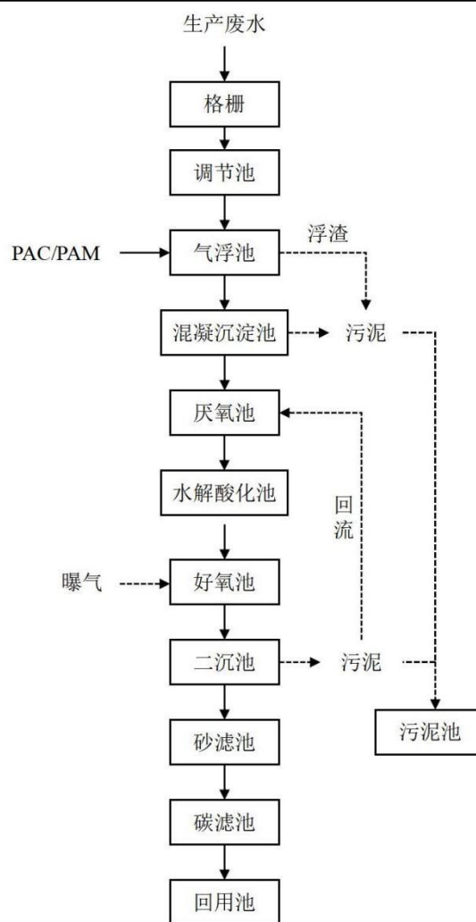
图 4-2 生产废水处理设施工艺流程图
