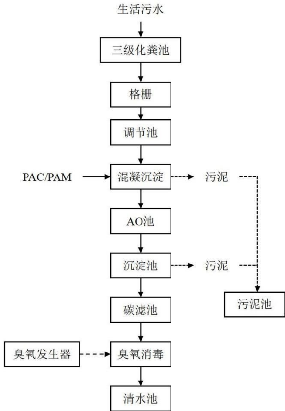
图 4-1 一体化生活污水处理设施工艺流程图
