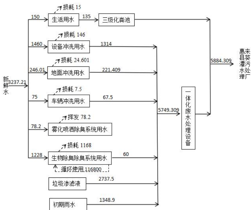
图2-1 厂区水平衡图 (t/a)
