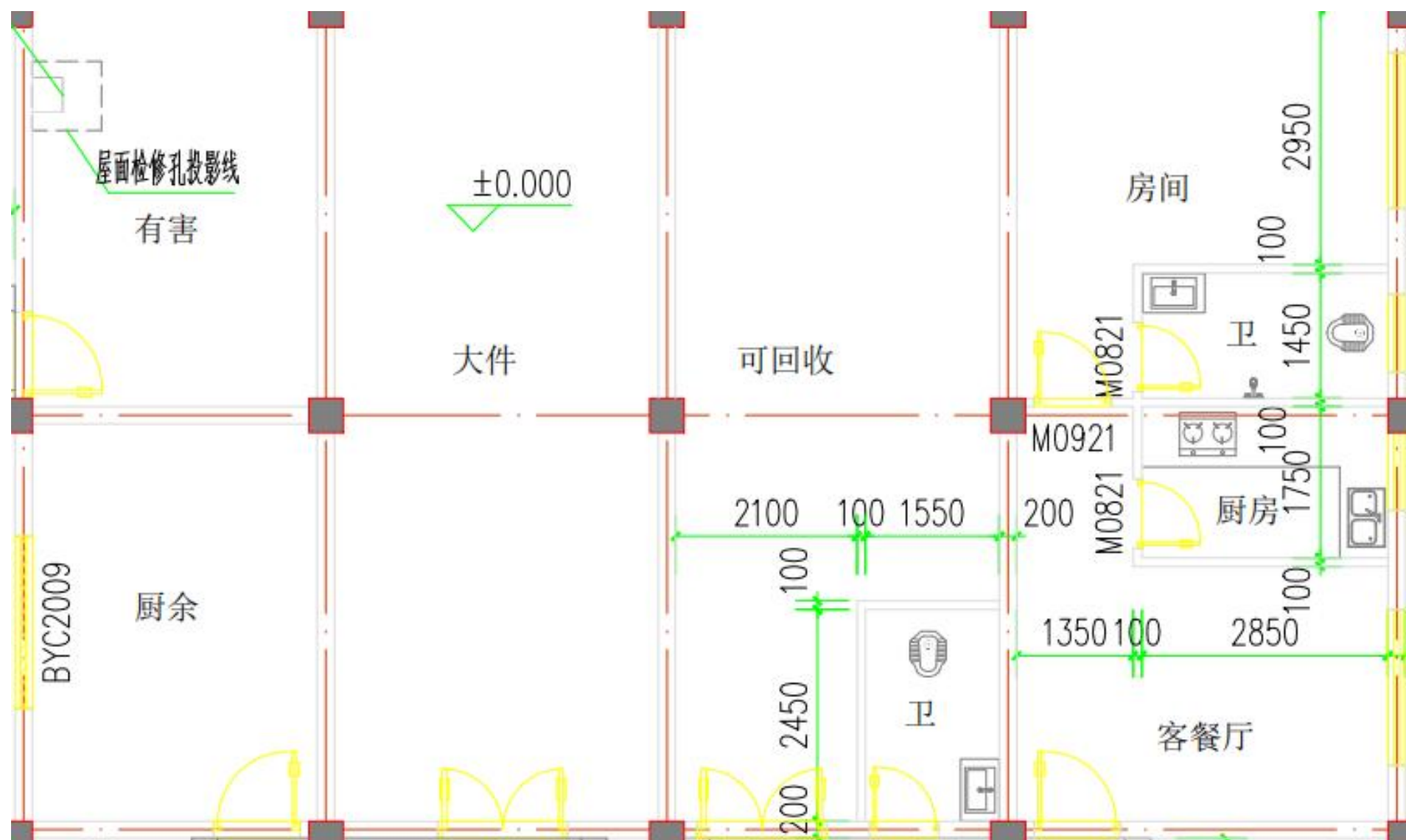
附图 2-3 项目平面布置图（配套房平面布置图）
