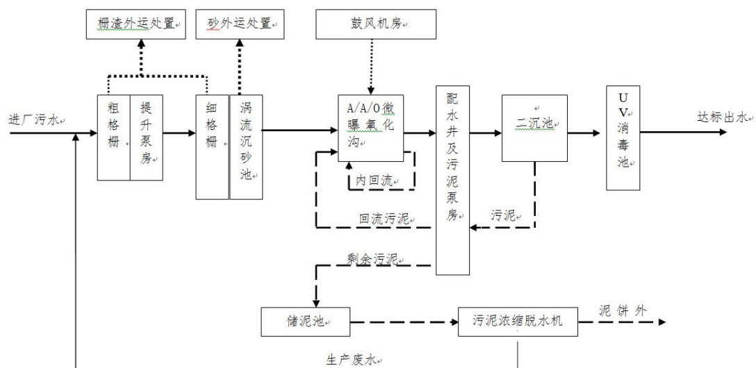
图 4-1 惠来县葵潭污水处理厂工艺流程图
