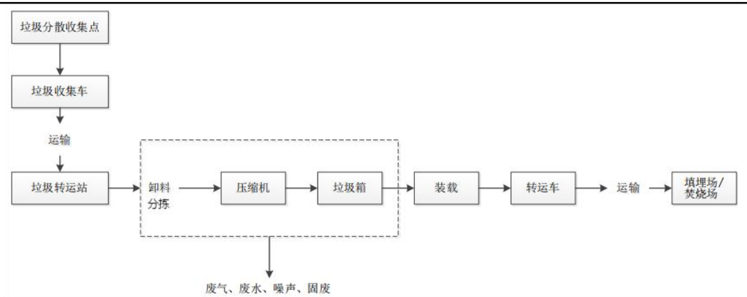
图2-3 项目工艺流程及产污环节图
