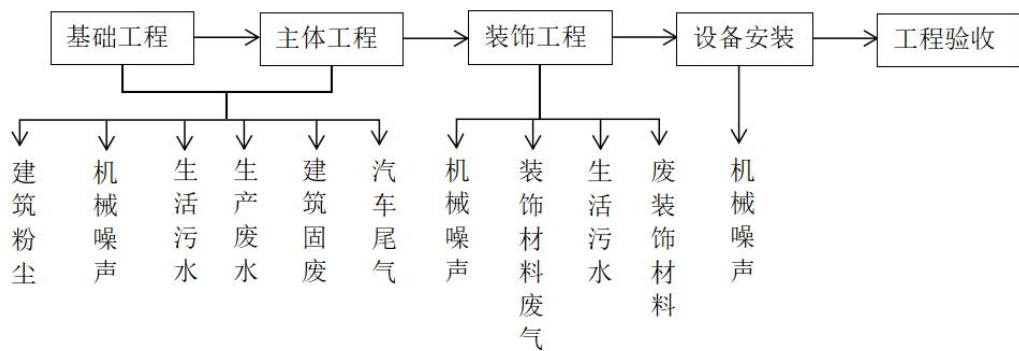
图2-2 项目施工期生产工艺流程及产污示意图
