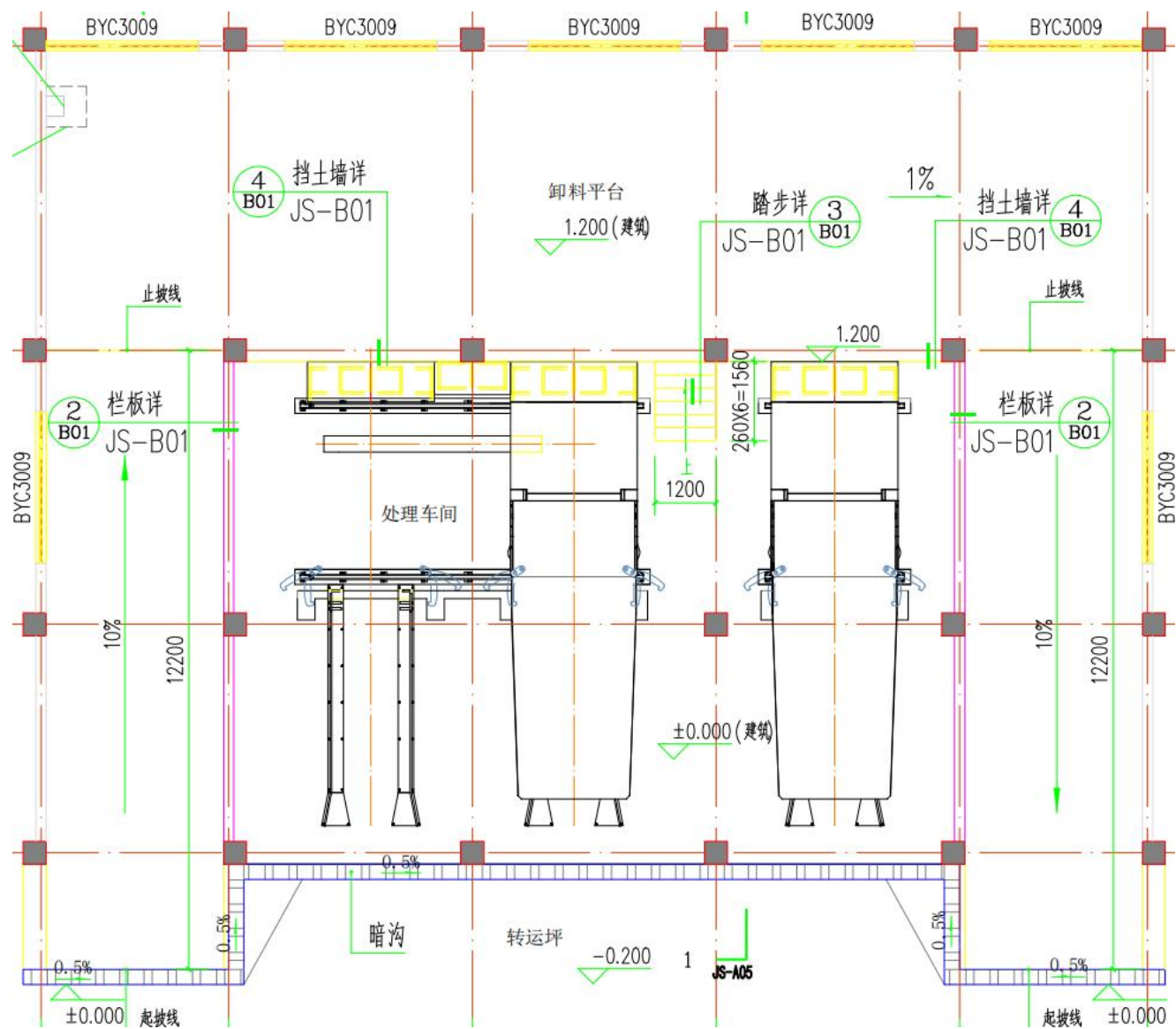
附图 2-2 项目平面布置图（压缩站车间平面布置图）
