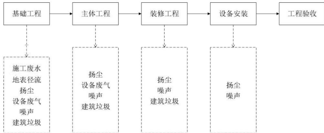
图2-3 施工期工艺流程及产污环节图
