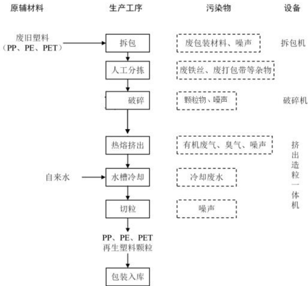
图 2-6 废旧塑料破碎-再生挤出造粒生产工艺流程及产污环节示意图
