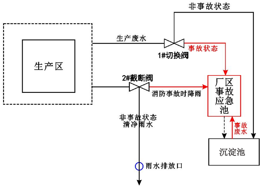
图 4-3 项目事故废水收集、封堵系统示意图
